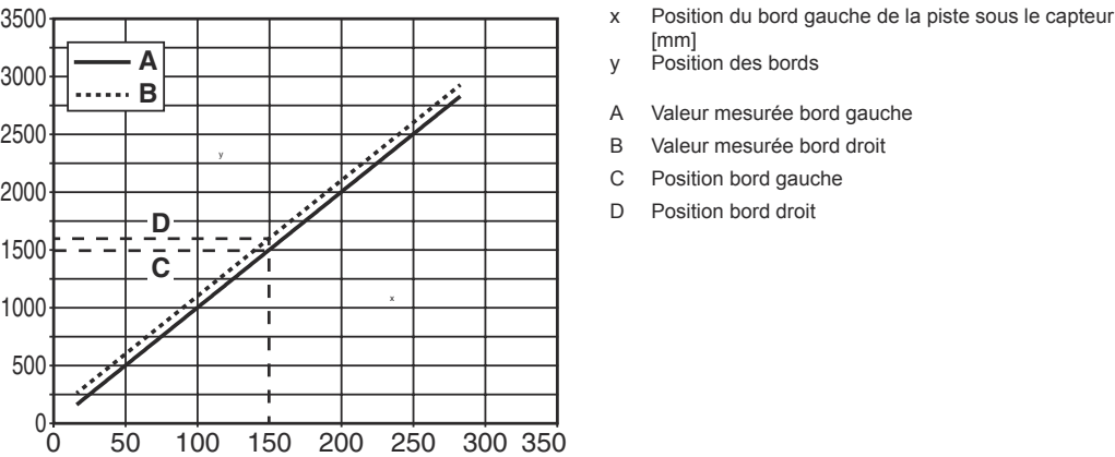
Courbe caractéristique du capteur avec une piste
