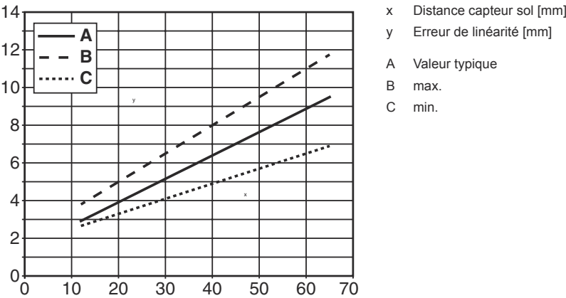
Courbe caractéristique du capteur avec une piste
