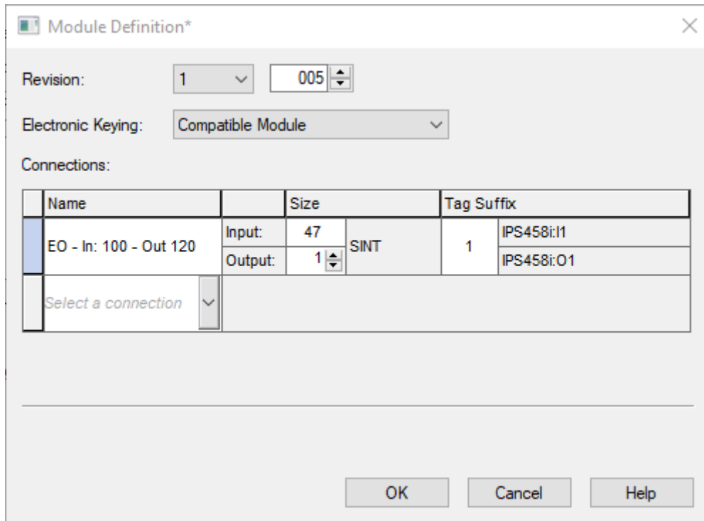
图 10.6: 配置示例 - 带 EDS 文件的模块定义
