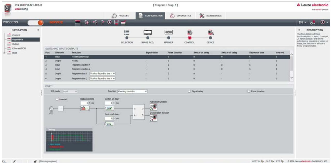
Fig. 9.8: E/S numériques
