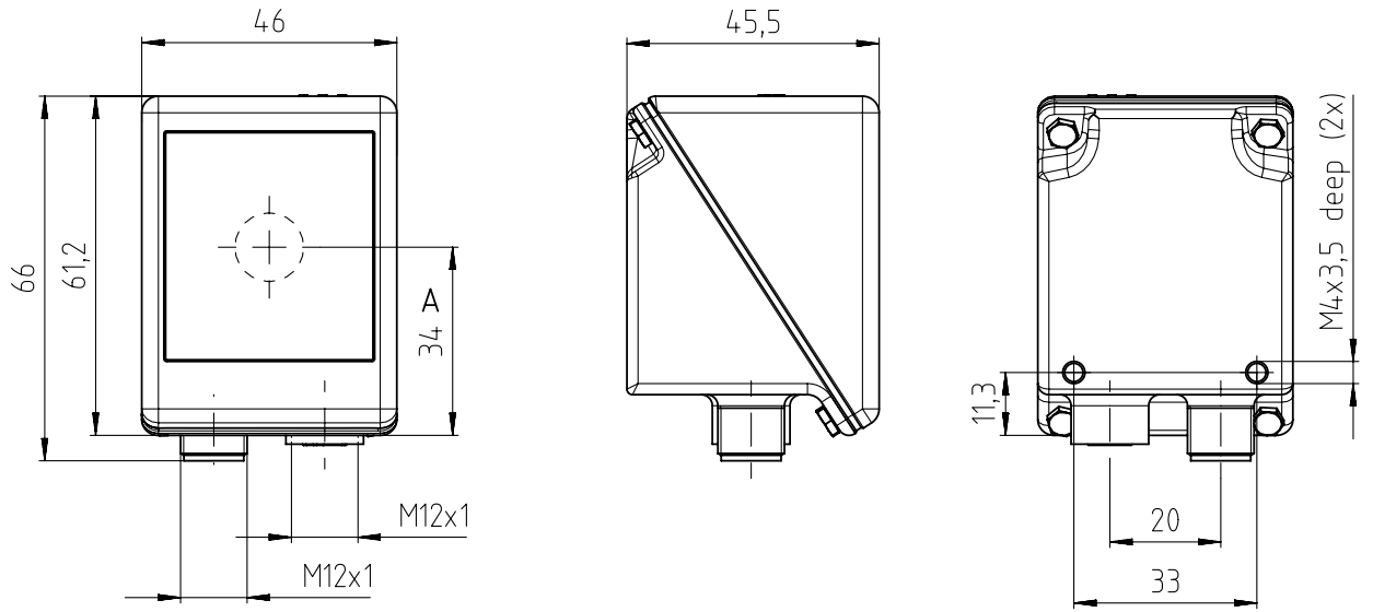
모든 치수(mm) A 광학 축 그림 15.2: 스테인리스 하우징이 있는 DCR 200i 치수 도면
