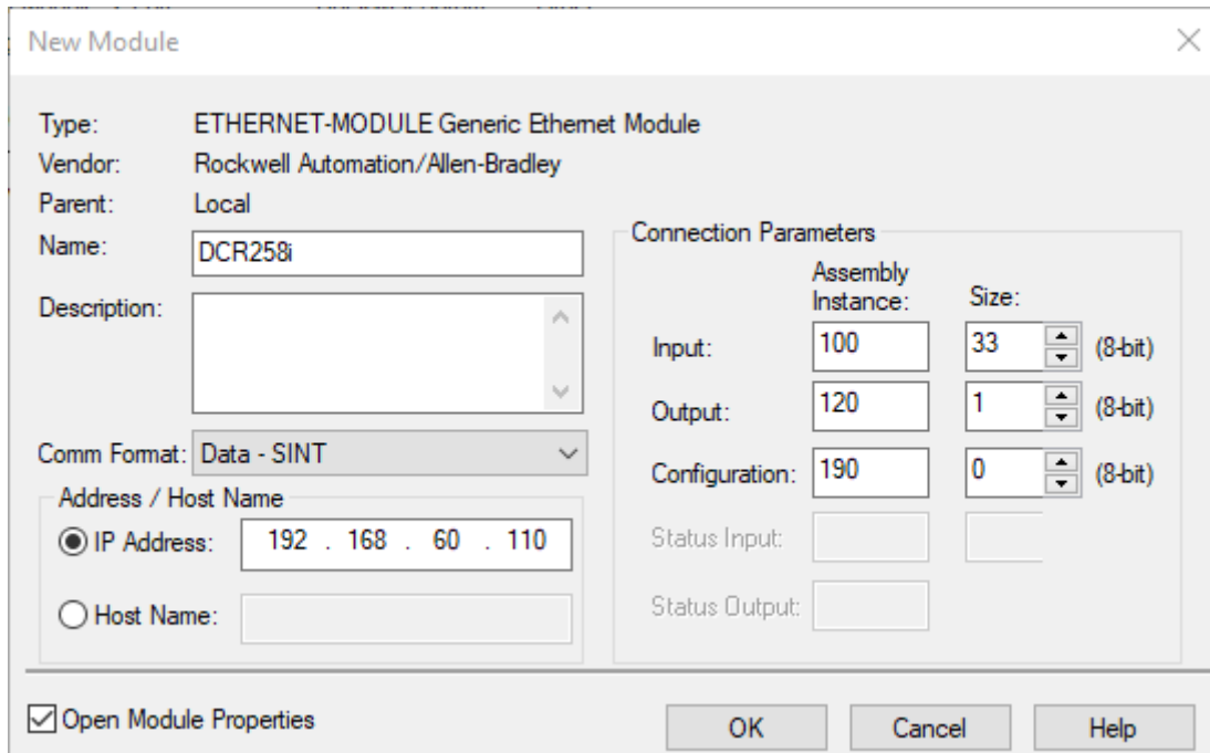
그림 10.2: Generic Ethernet Module 대화상자
