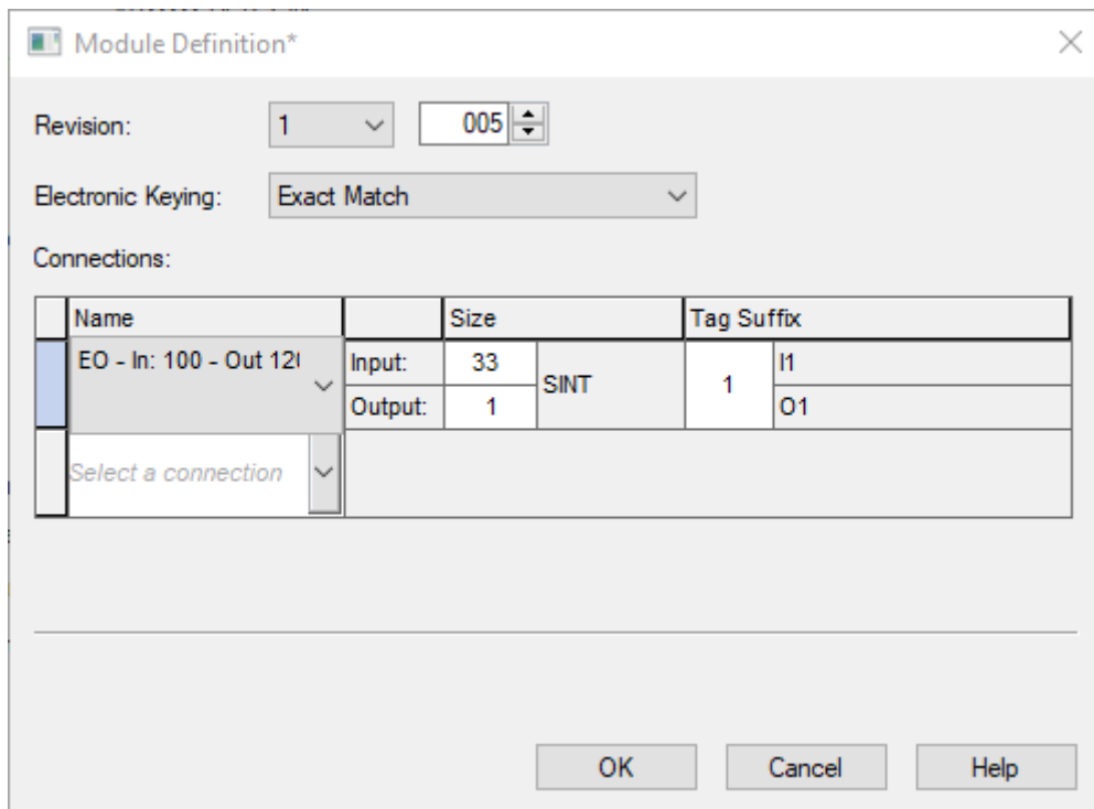
그림 10.6: 설정 예시 – EDS 파일을 이용한 모듈 정의
