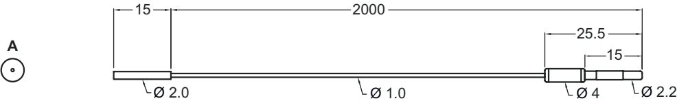
A Ø 0.25 mm 光ファイバーコア x 1個
