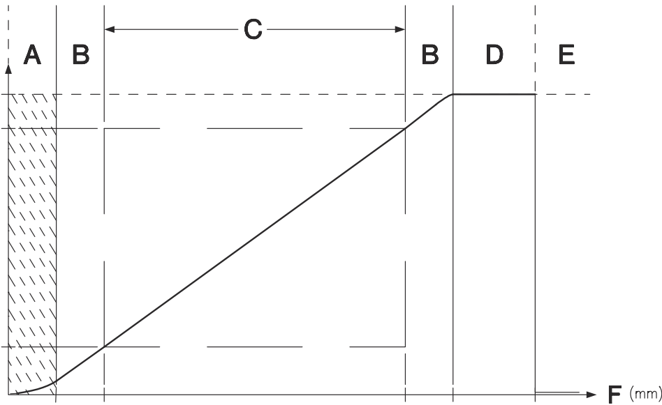
Charakterystyka wyjściowa wyjścia analogowego
