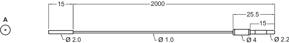
A Ø 0.25 mm 玻璃纤维芯 x 1 件
