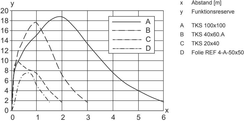
Typ. Funktionsreserve
