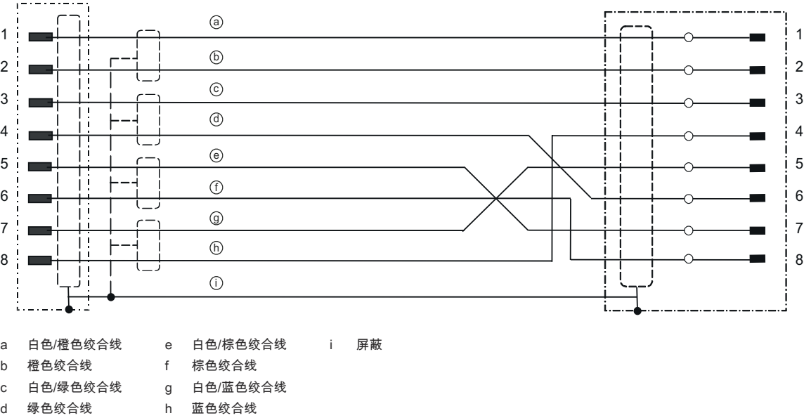
接线图
