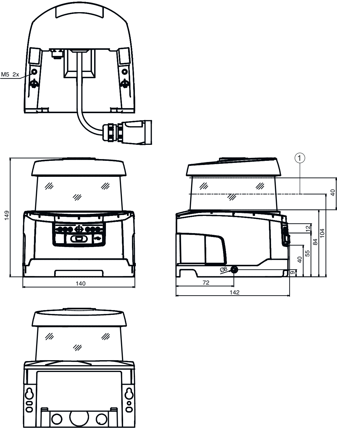
1 扫描平面
