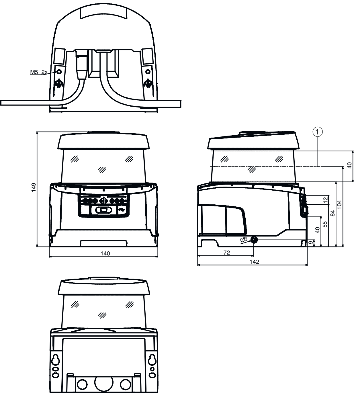
1 扫描平面
