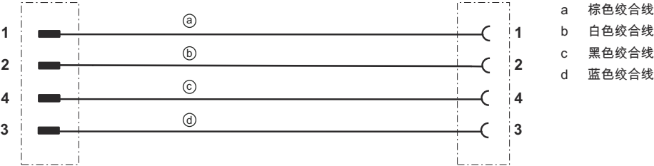
接线图
