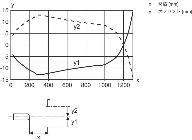
典型的応答挙動 ( 調整距離 1300mm )
