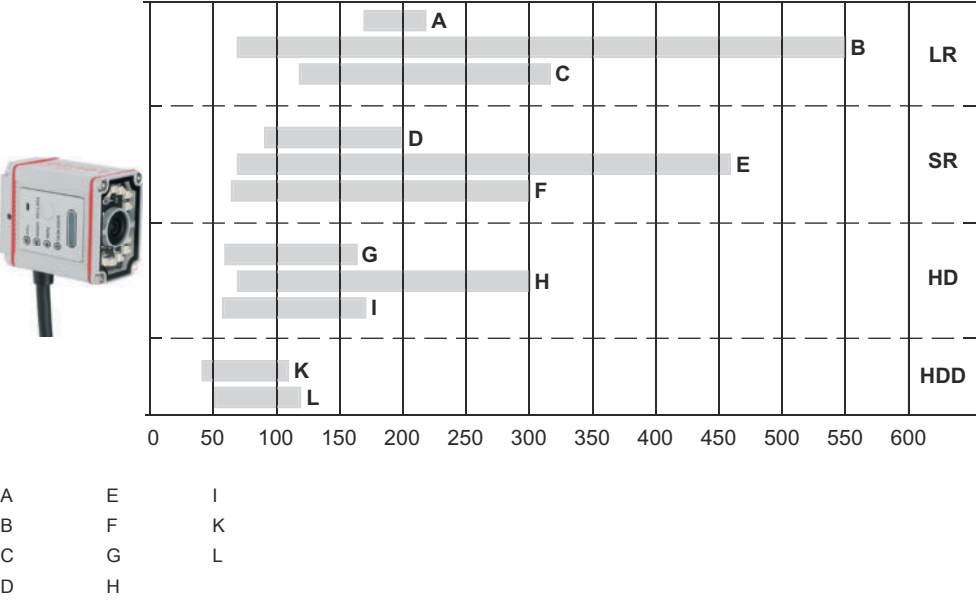
读取距离 ( 典型 )
