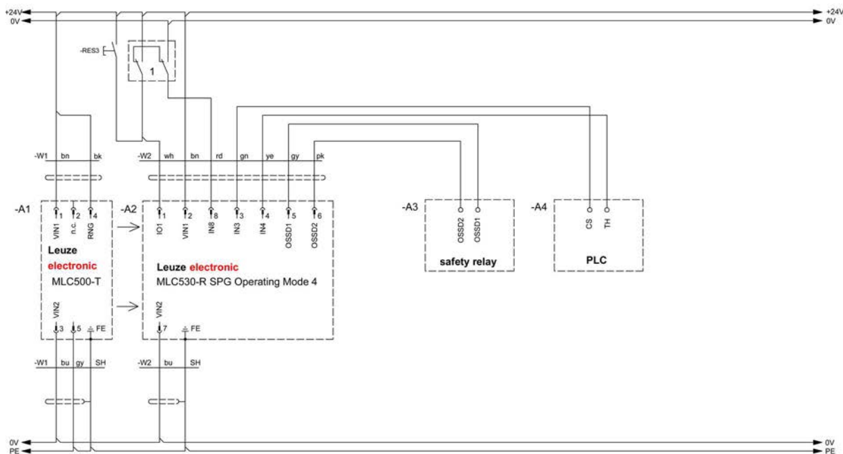
Fig. 8.5: Mode de fonctionnement 4 : exemple de câblage avec Smart Process Gating (SPG)
