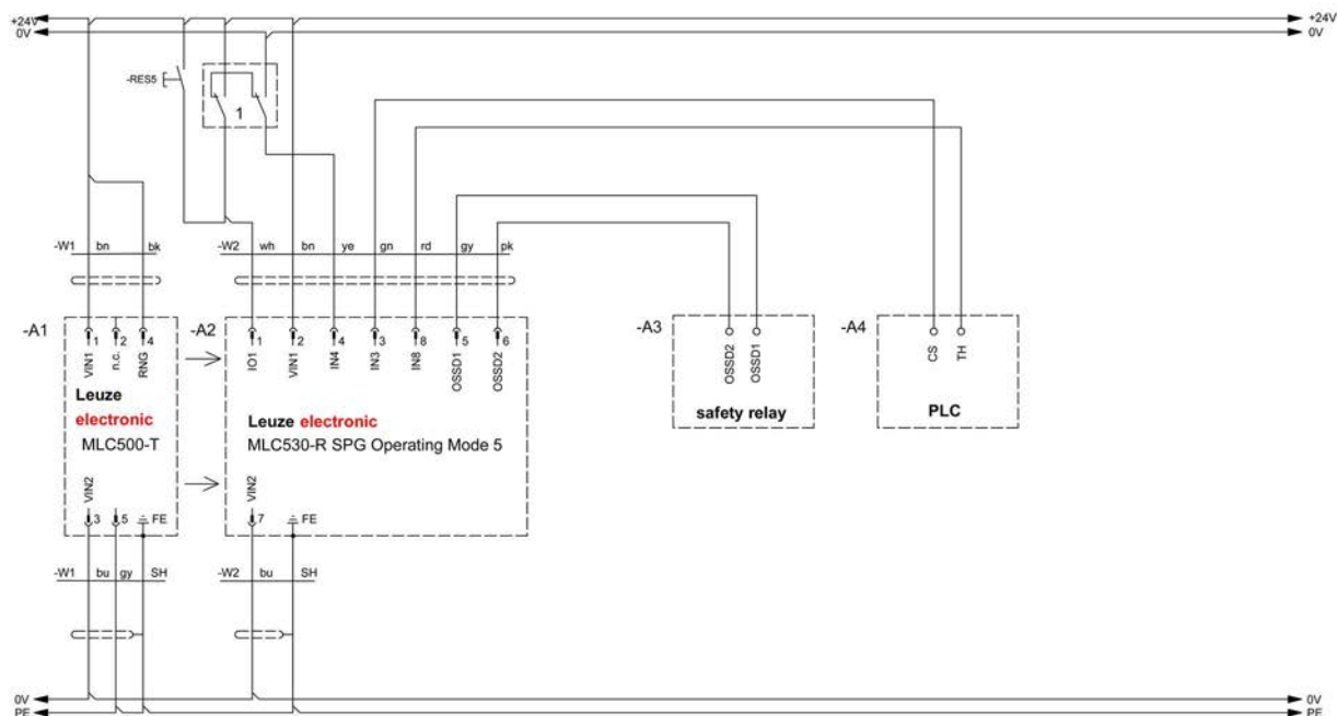
Fig. 8.6: Mode de fonctionnement 5 : exemple de câblage avec Smart Process Gating (SPG)
