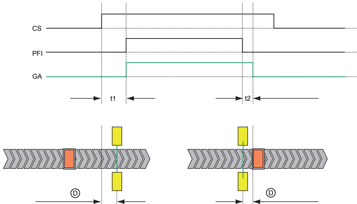
Fig. 4.1: Principe du SPG
