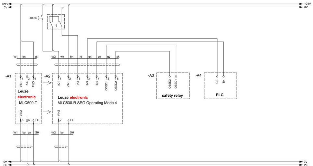
Figura 8.5: Modo de trabajo 4: ejemplo de circuito con Smart Process Gating (SPG)
