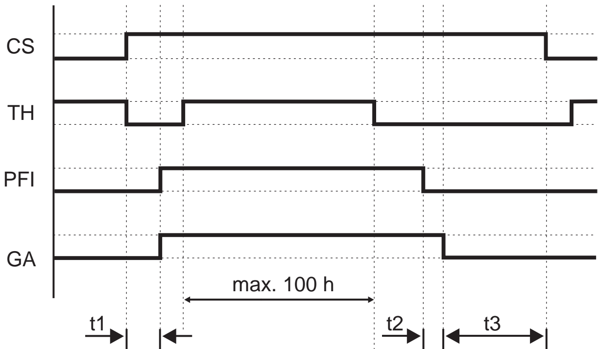
Figura 4.9: Prolongación del timeout de SPG
