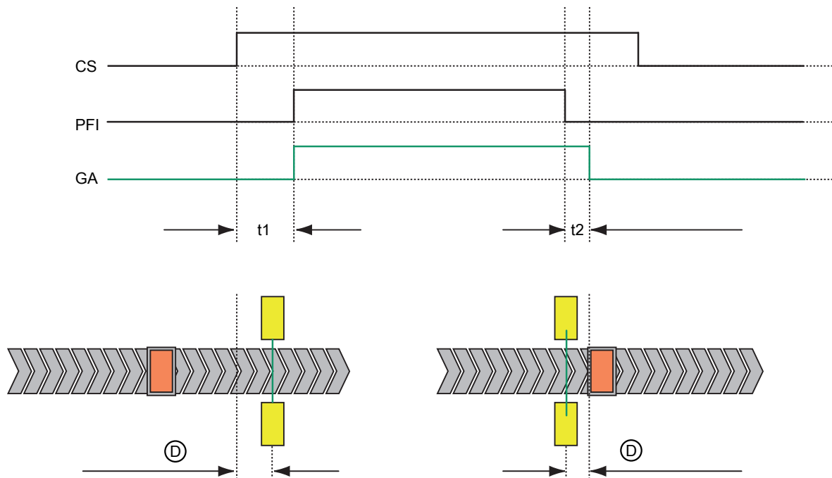
Figura 4.1: Principio SPG
