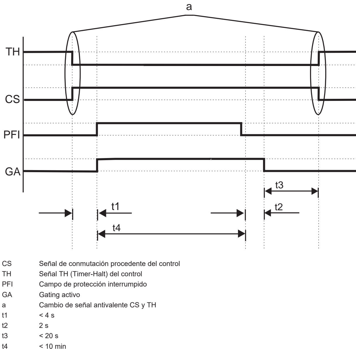
Figura 4.2: Modo de trabajo 1 - Stop cualificado
