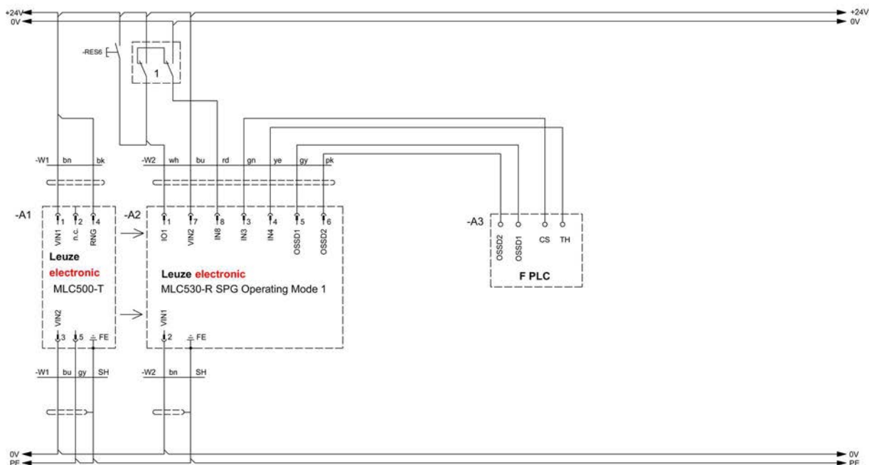
Figura 8.4: Modo de trabajo 1: ejemplo de conexión con Smart Process Gating (SPG)
