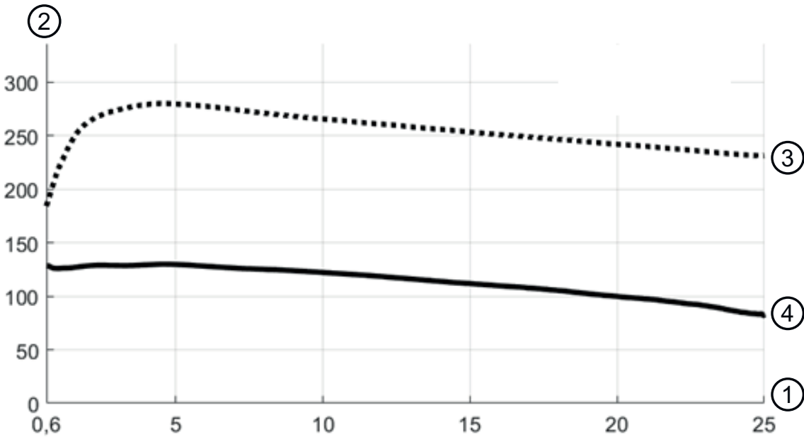
1 물체 거리[m] 2 신호 세기 3 역반사판 비닐랩 4 흰색 표면 그림은 안전센서가 전송한 신호 세기의 전형적인 경과를 다음 경계 조건에서 측정된 물체 거리 및 물체 확산 반사에 따라
