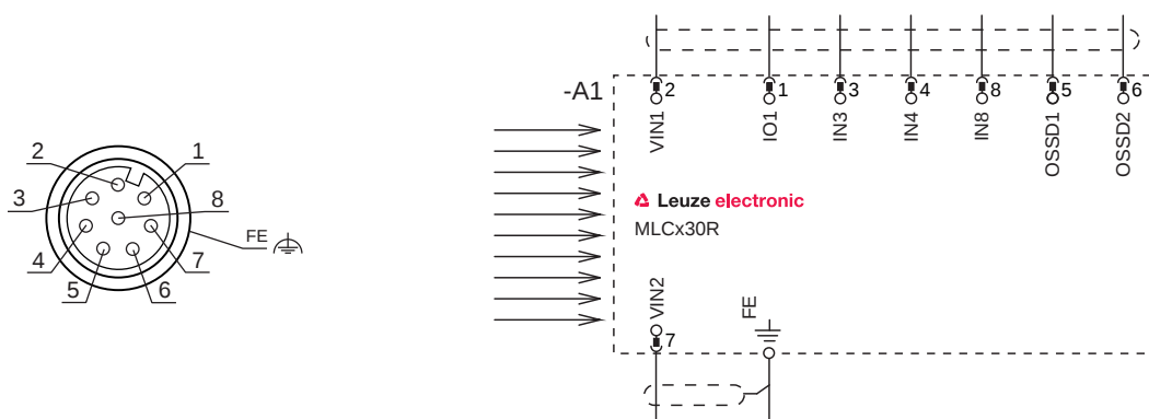
Figura 8.3: Asignación de conector y esquema de conexiones del receptor
