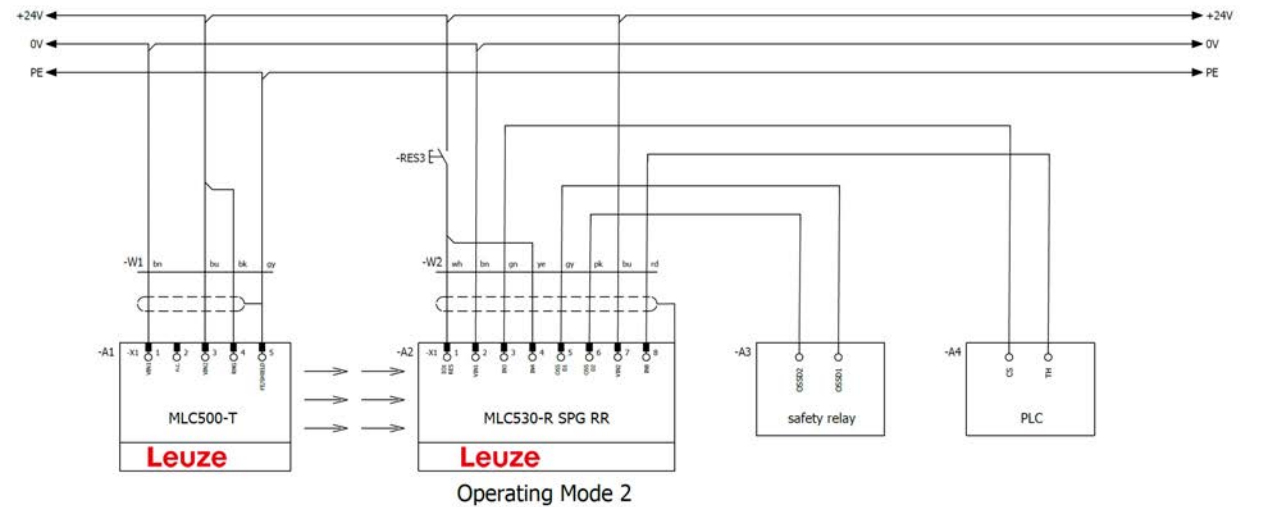
Figura 8.32: Modo de funcionamiento 2: ejemplo de circuito con Smart Process Gating (SPG)
