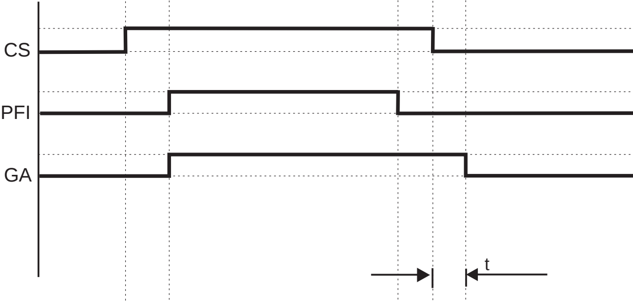
Figura 4.12: Final de gating controlado en los modos de funcionamiento 4 y 5
