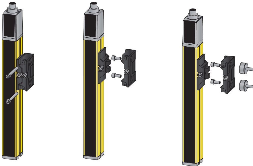
Figura 7.9: Montaje a través de soporte orientable BT-2SB10
