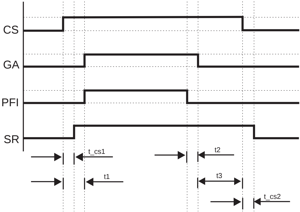
Figura 4.9: Modo de funcionamiento 4
