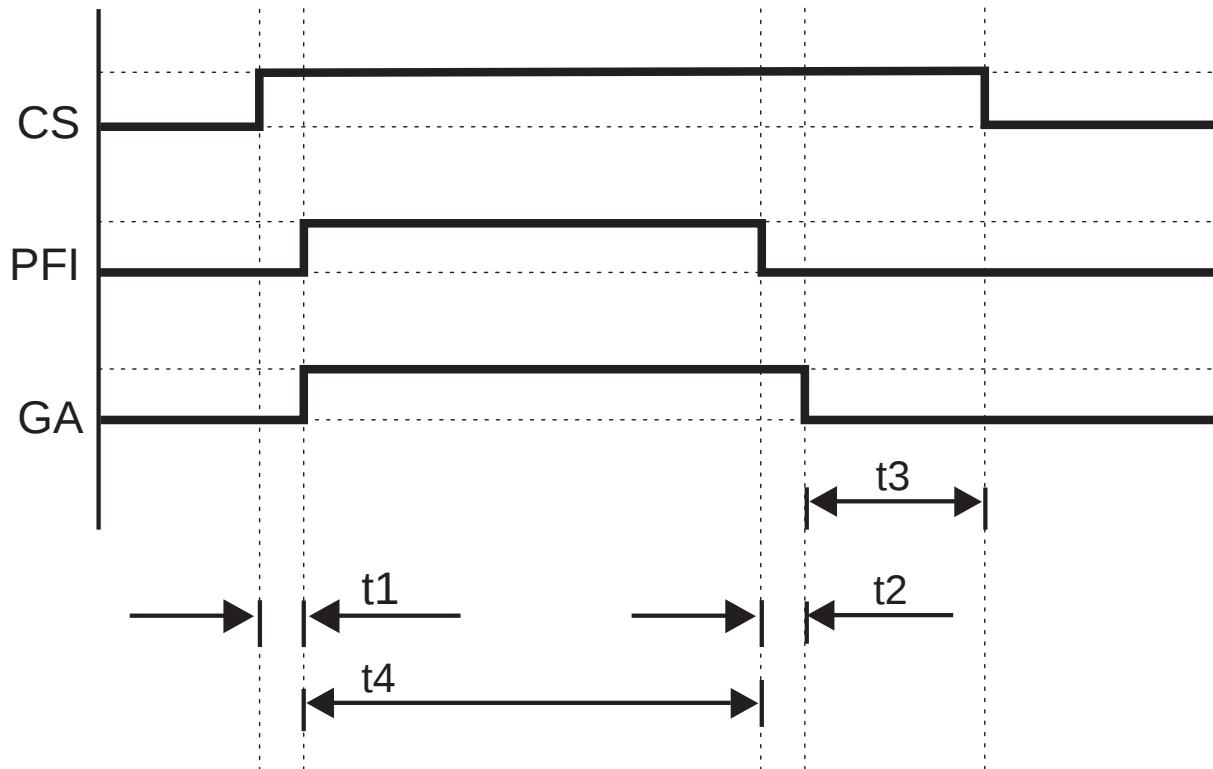
Figura 4.11: Modo de funcionamiento 6
