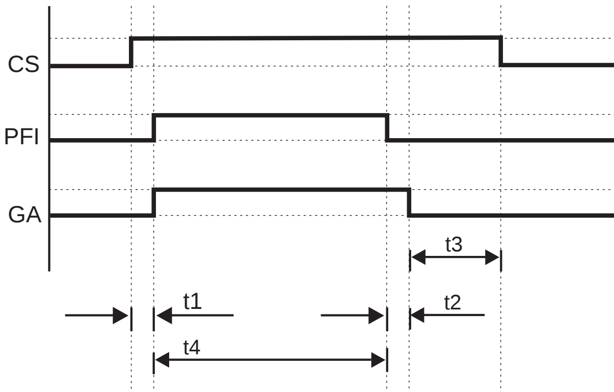
Figura 4.7: Modo de funcionamiento 2
