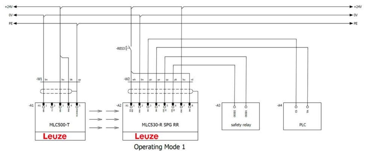
Figura 8.31: Modo de funcionamiento 1: ejemplo de conexión con Smart Process Gating (SPG)
