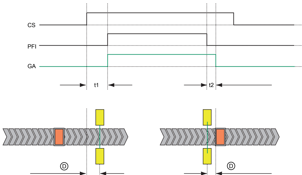
Figura 4.1: Principio SPG
