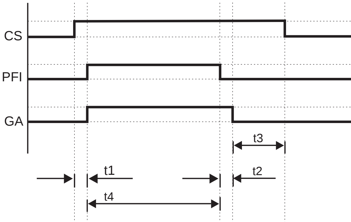
Figura 4.10: Modo de funcionamiento 5
