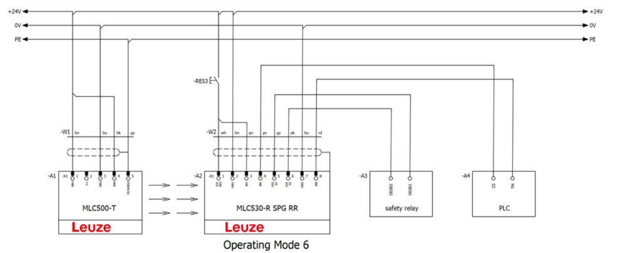
Figura 8.36: Modo de funcionamiento 6: ejemplo de circuito con Smart Process Gating (SPG)
