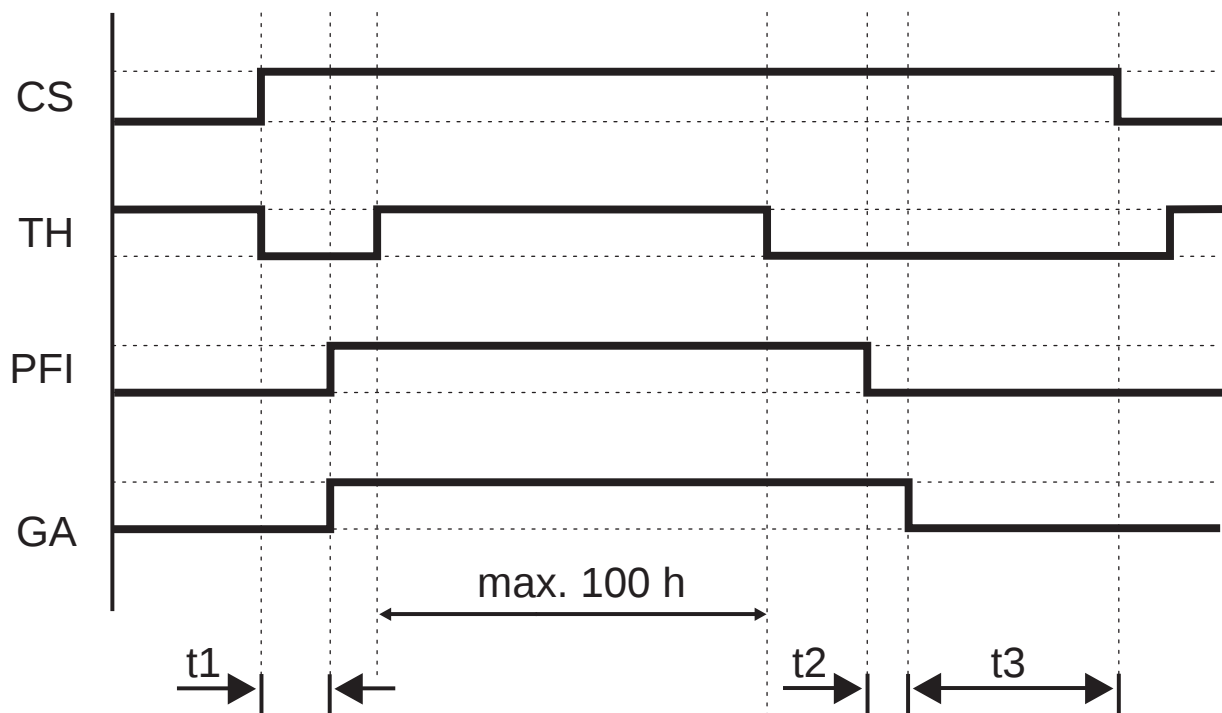
Figura 4.4: Prolongación del timeout de SPG
