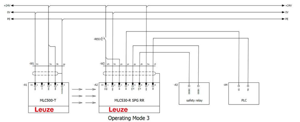
Figura 8.33: Modo de funcionamiento 3: ejemplo de circuito con Smart Process Gating (SPG)
