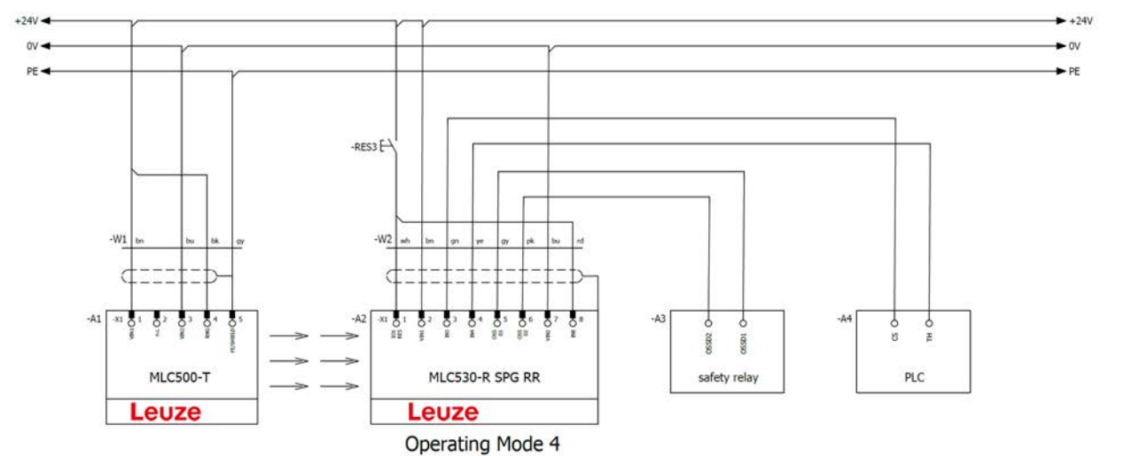
Figura 8.34: Modo de funcionamiento 4: ejemplo de circuito con Smart Process Gating (SPG)
