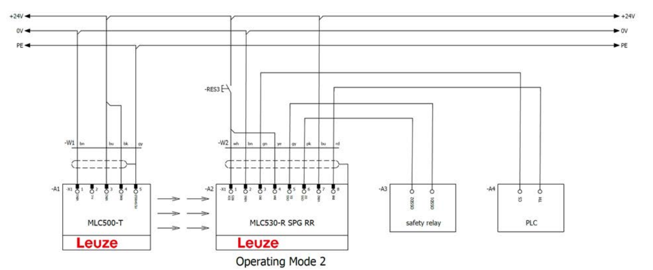
图 8.32: 运行模式 2：含智能过程门控 (SPG) 的接线示例
