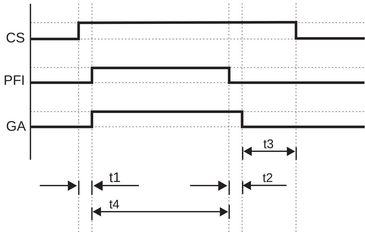
图 4.7: 运行模式 2 CS 控制系统的控制信号 PFI 保护区域中断 GA 门控激活 t1 < 4 s t2 1 s t3 < 20 s t4 < 10 分钟
