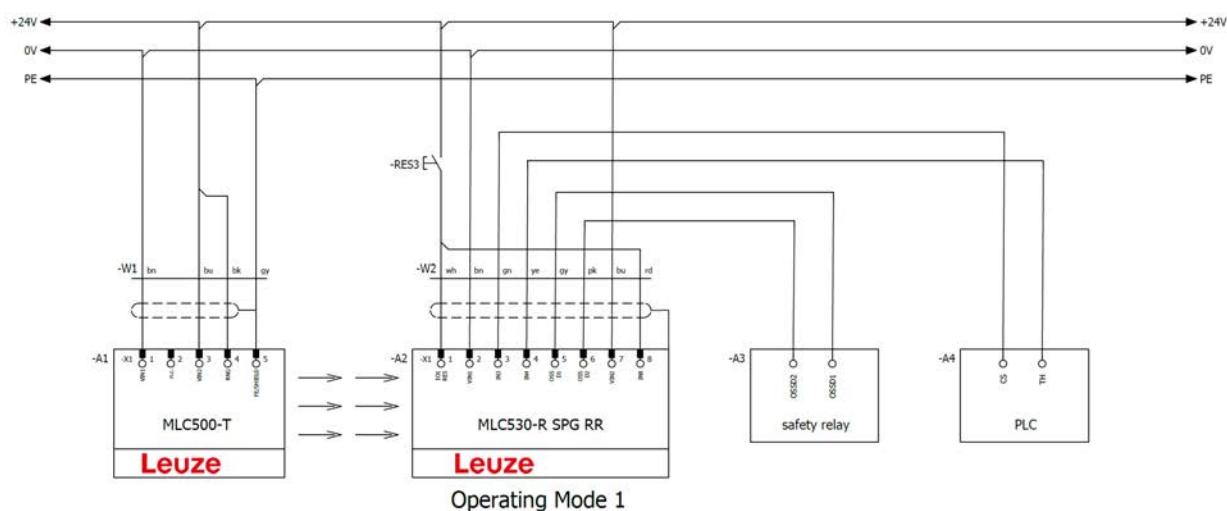
图 8.31: 运行模式 1：含智能过程门控 (SPG) 的连接示范
