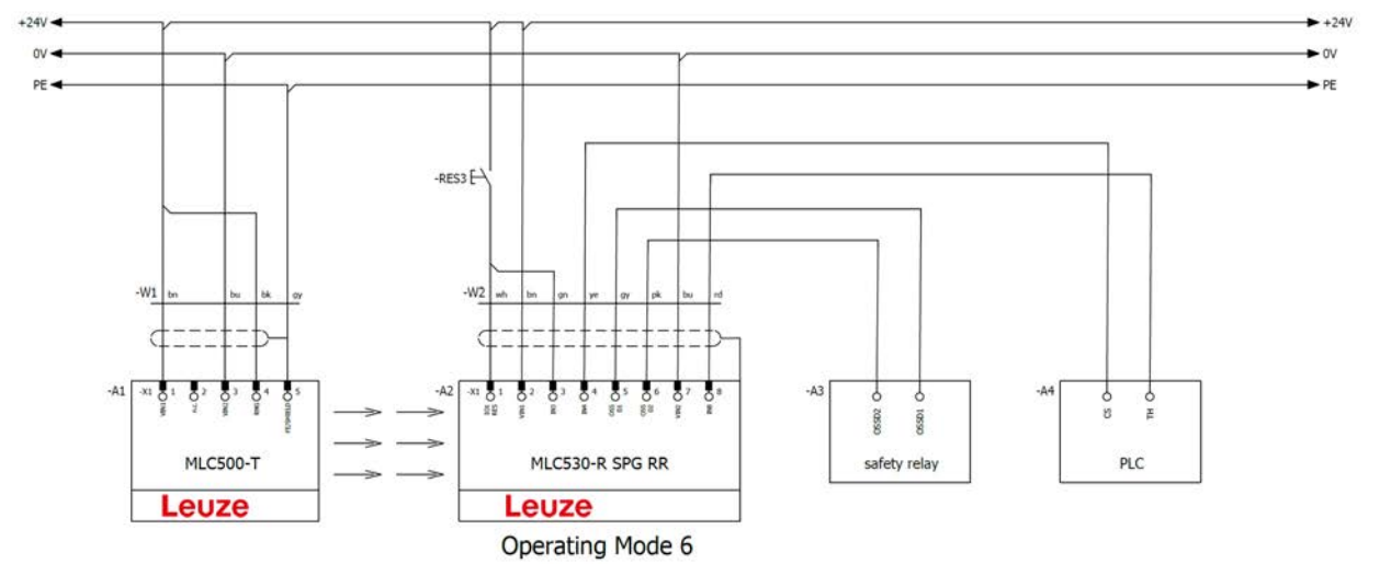
图 8.36: 运行模式 6：含智能过程门控 (SPG) 的接线示例
