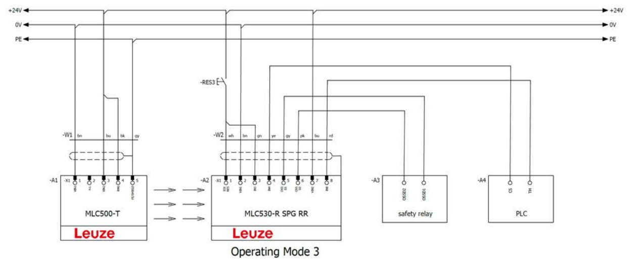
图 8.33: 运行模式 3 : 含智能过程门控 (SPG) 的接线示例
