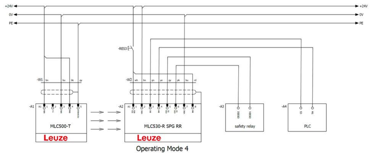
图 8.34: 运行模式 4 : 含智能过程门控 (SPG) 的接线示例
