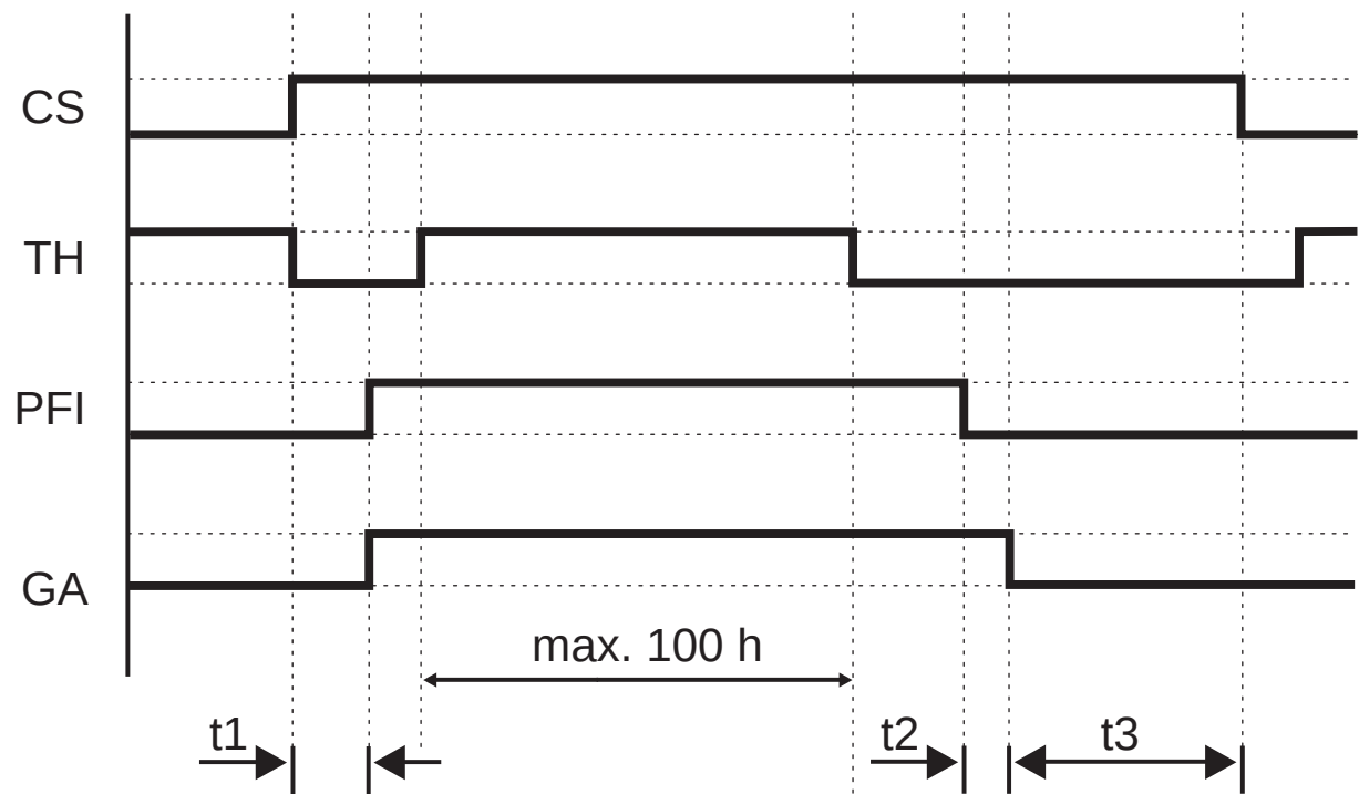
图 4.4: SPG 限定时间延长 CS 控制系统的控制信号 TH 控制系统的定时器中断信号 PFI 保护区域中断 GA 门控激活 t1 < 4 s t2 1 s t3 < 20 s
