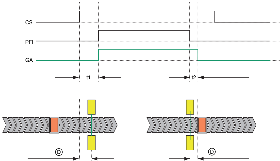
图 4.1: SPG 原理 CS 控制系统的控制信号 PFI 保护区域中断 GA 门控激活 t1 < 4 s t2 1 s D < 200 mm
