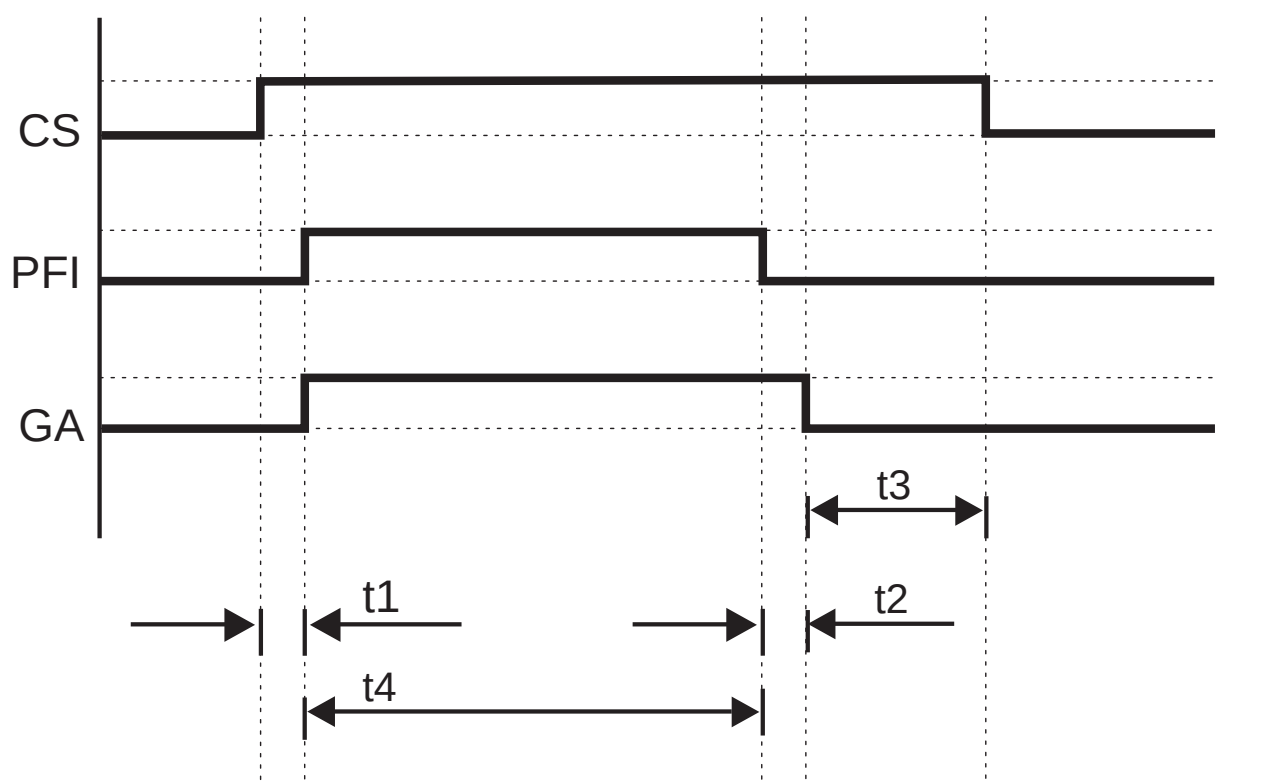
图 4.11: 运行模式6 CS 控制系统的控制信号 PFI 保护区域中断 GA 门控激活 t1 < 4 s t2 1 s t3 < 20 s t4 <10分钟
