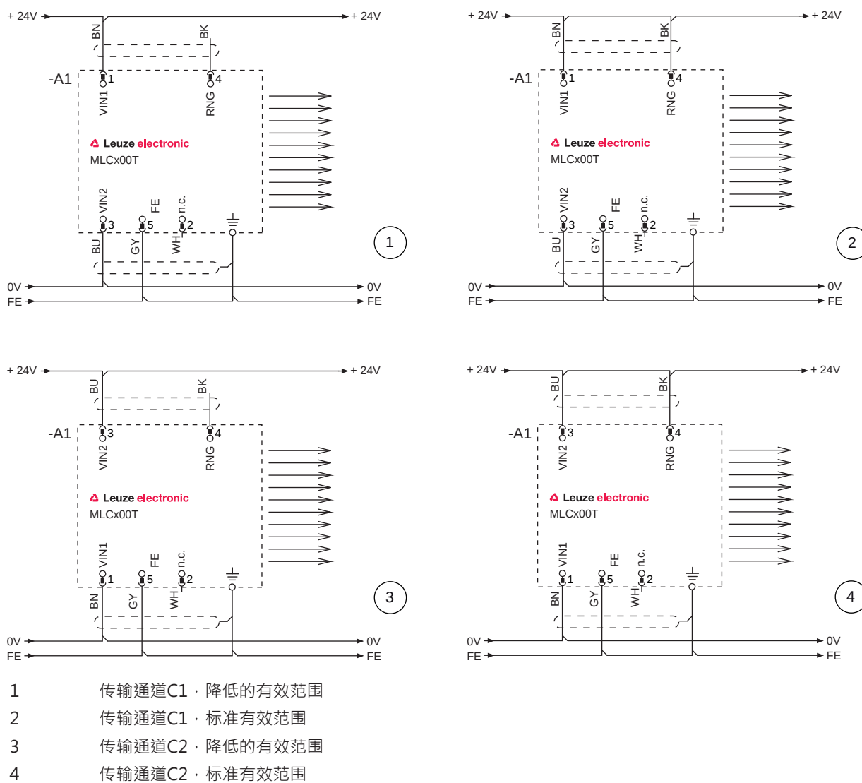
图 8.2: 发射器连接示例
