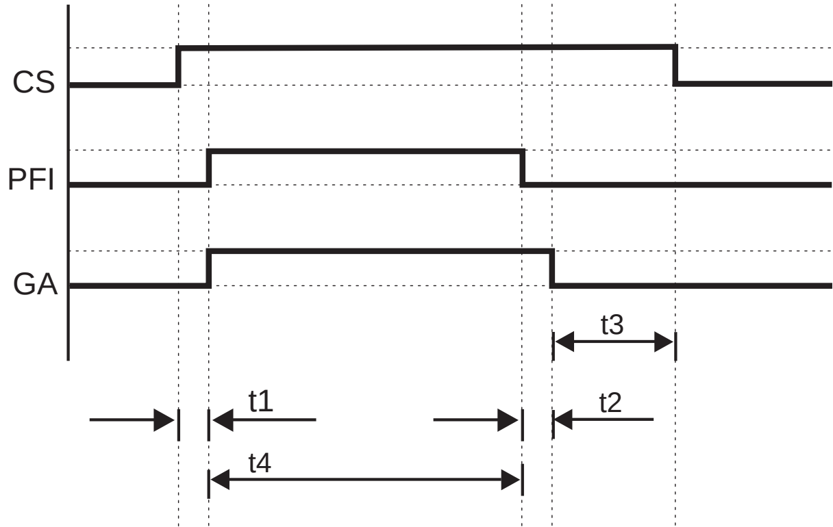
图 4.10: 运行模式5 CS 控制系统的控制信号 PFI 保护区域中断 GA 门控激活 t1 < 4 s t2 1 s t3 < 20 s t4 <10分钟
