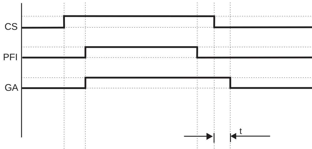
图 4.12: 运行模式 BA 4 和 BA 5 中受控结束门控
