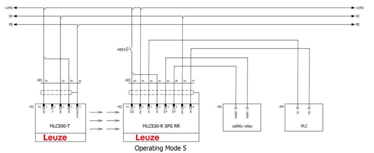
图 8.35: 运行模式 5：含智能过程门控 (SPG) 的接线示例
