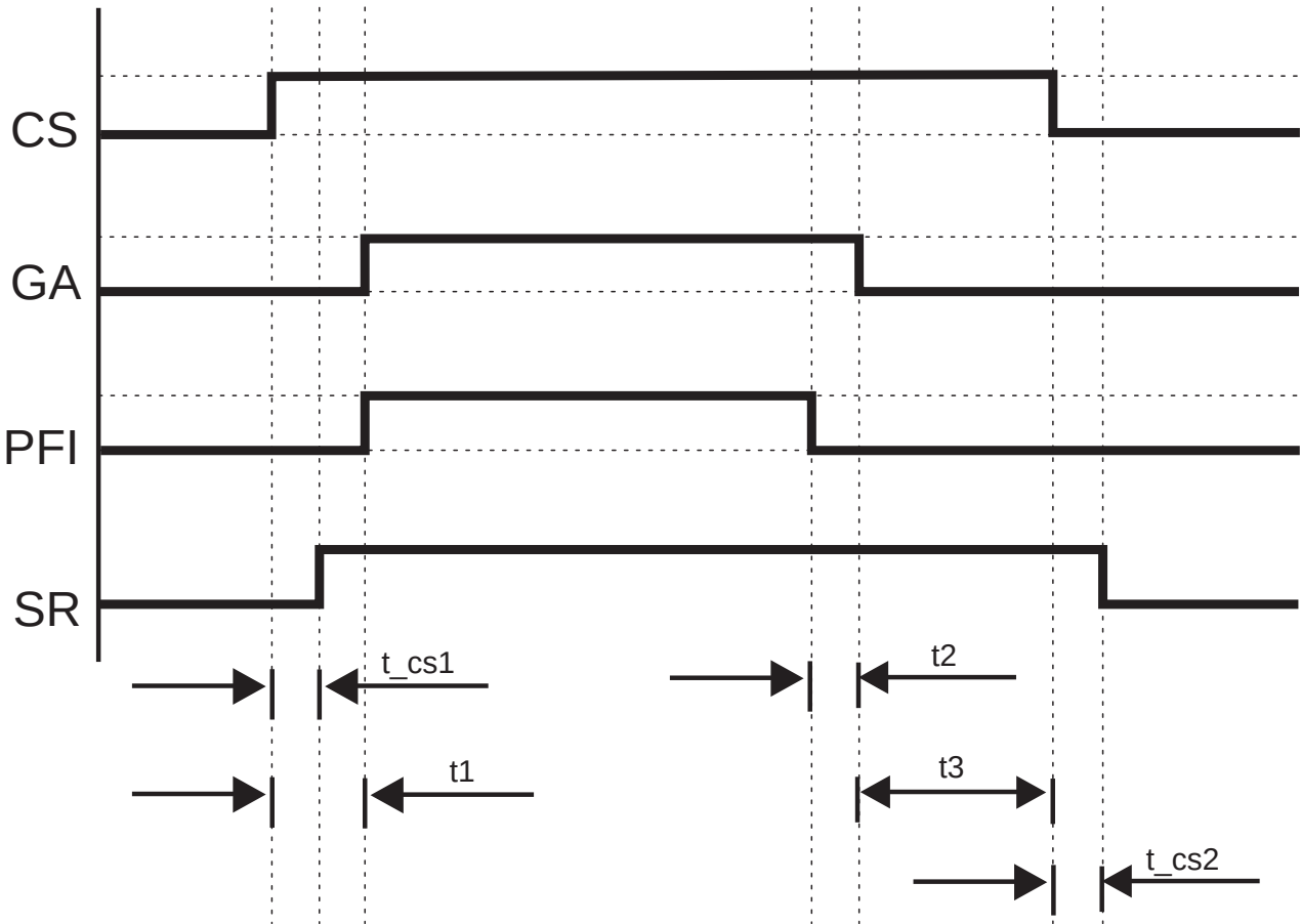
图 4.9: 运行模式4
