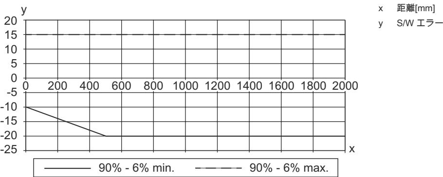
S/W エラーダイアグラム
