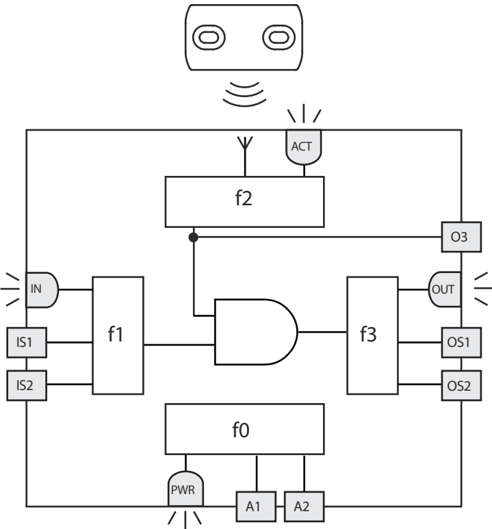
Diagrama de conexões interno
