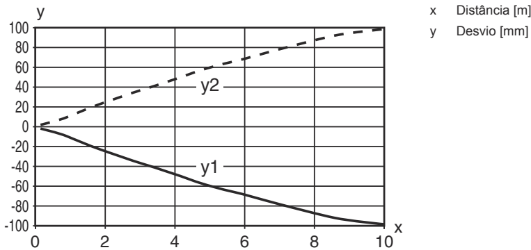
Comportamento de resposta típ. (TKS100x100)
