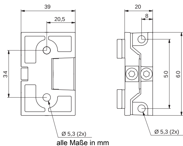
Bild 20.8: Schwenkhalterungen BT-2SB10/BT-2SB10-S
