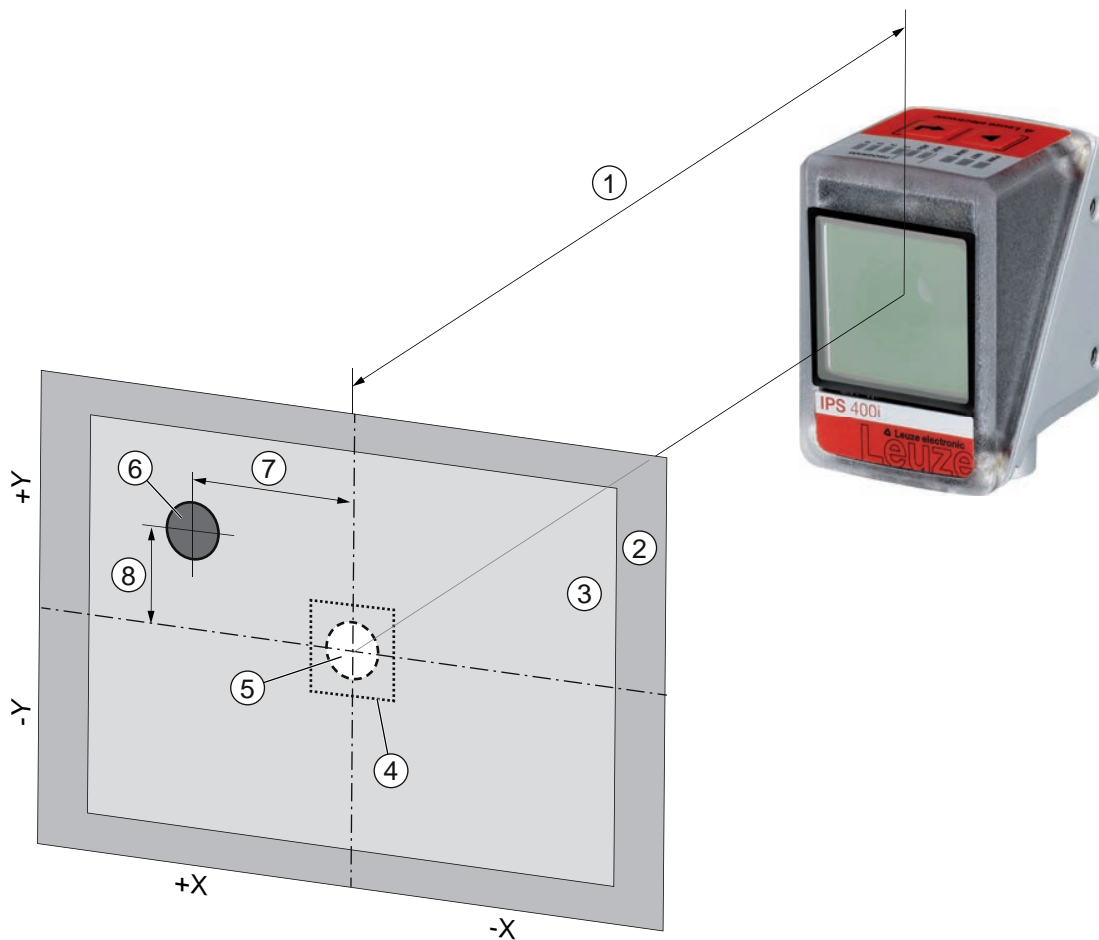
Bild 4.1: Arbeitsweise des Positionierungssensors
