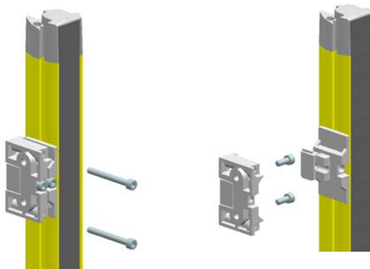
图 5.7: 使用旋转支架 BT-2SB05 和 M5 螺钉安装
