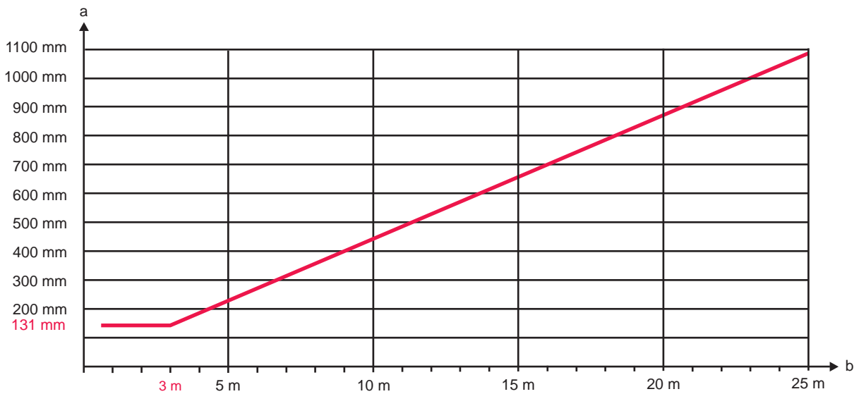
图 5.2: 根据保护区的宽度决定的与反射平面的最小距离
