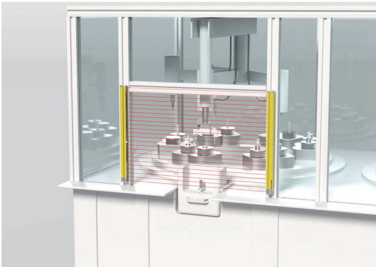
图 4.1: 操作保护点
