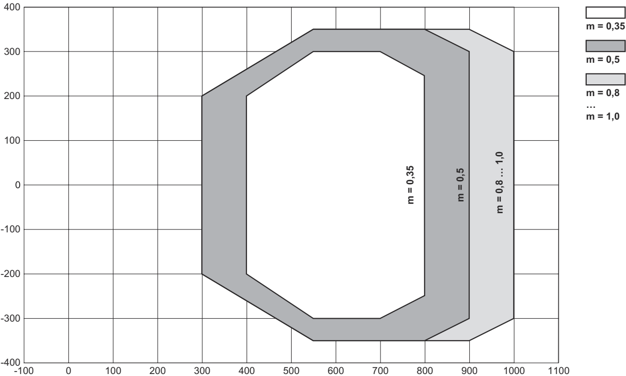
Curva del campo di lettura
