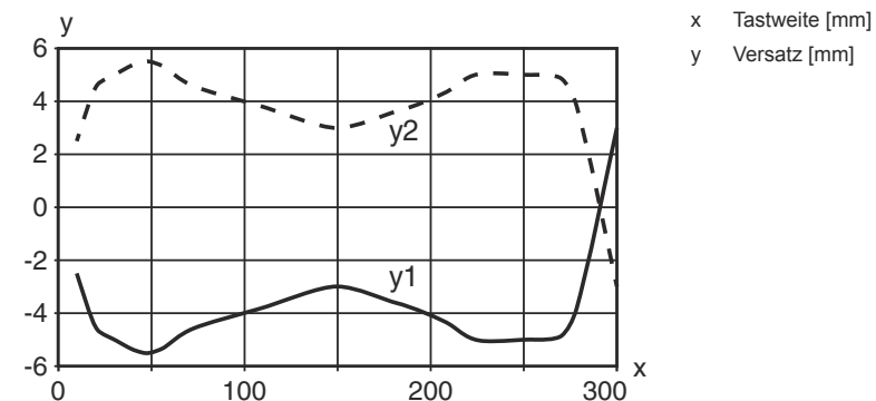
Typ. Ansprechverhalten (Einstellentfernung 300 mm)
