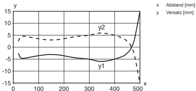
Typ. Ansprechverhalten (Einstellentfernung 500 mm)
