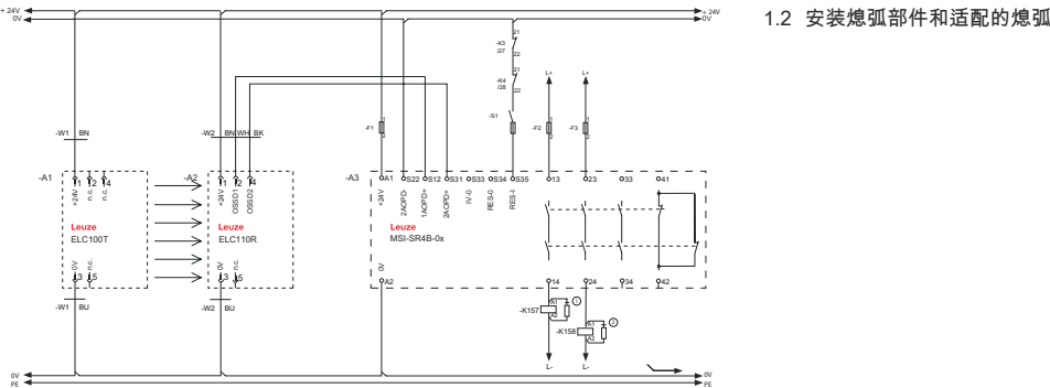
带后置安全控制器MSI-SR4B的接线示例
