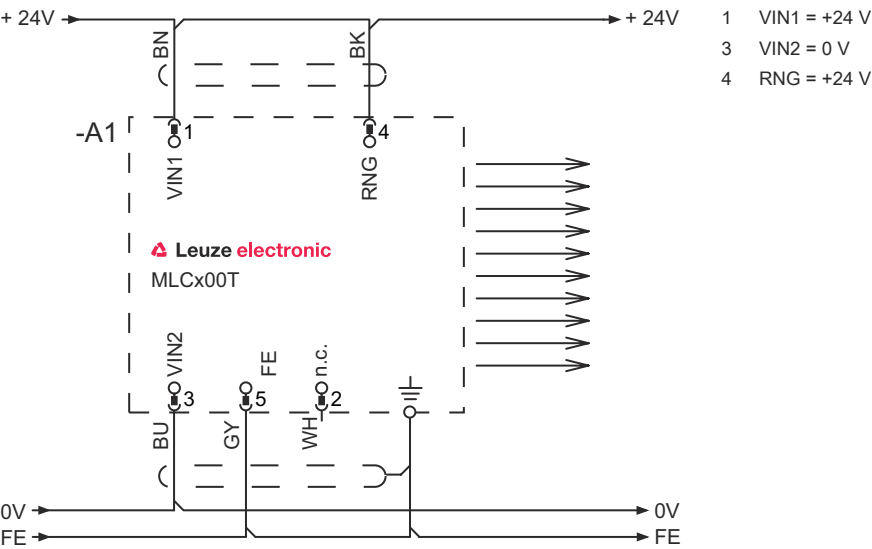
传输通道 C1，接收器上的 OSSD 已激活
