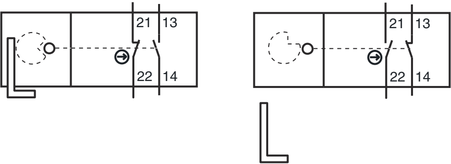
21/22 强制常闭触点 (NC)
