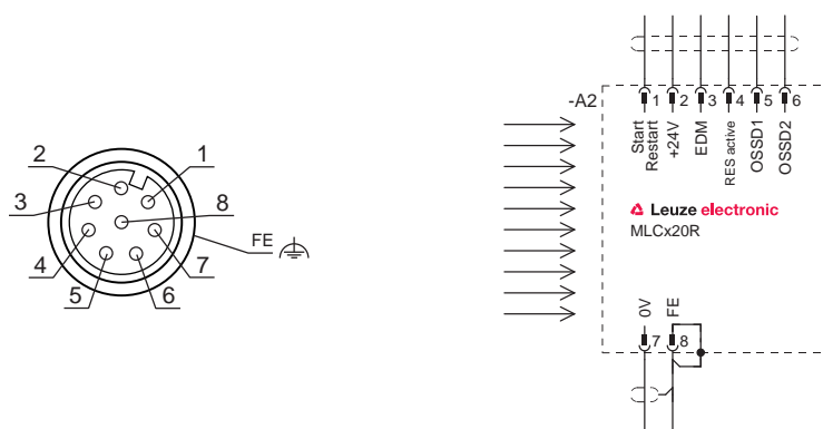
Figura 7.4: Occupazione dei pin e schema di collegamento del ricevitore
