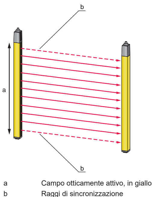
Figura 3.1: Sistema trasmettitore-ricevitore
