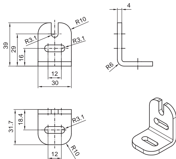
Fig. 14.2: Support équerre BT-L
