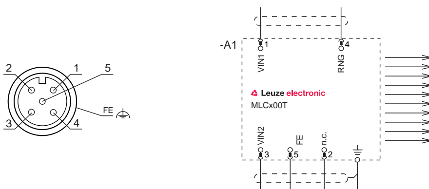
Figura 7.2: Asignación de conector y esquema de conexiones del emisor
