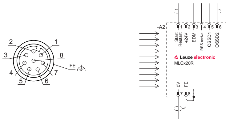
Figura 7.4: Asignación de conector y esquema de conexiones del receptor
