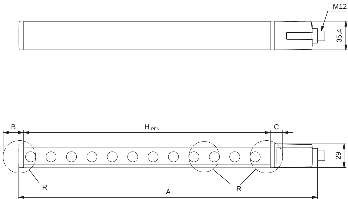
图 14.1: 发射器和接收器尺寸 有效保护高度 H_{PFE} 超过光学范围，到达R圆的外缘。 计算有效保护高度
