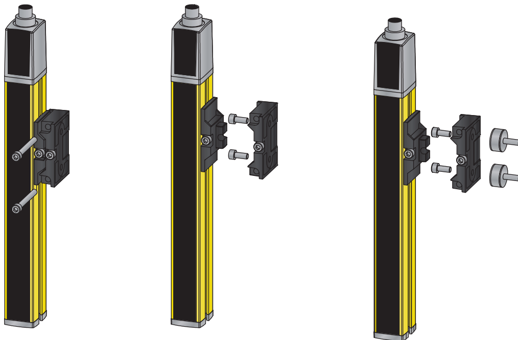
Fig. 6.9: Montagem através de suportes orientáveis BT-2SB10
