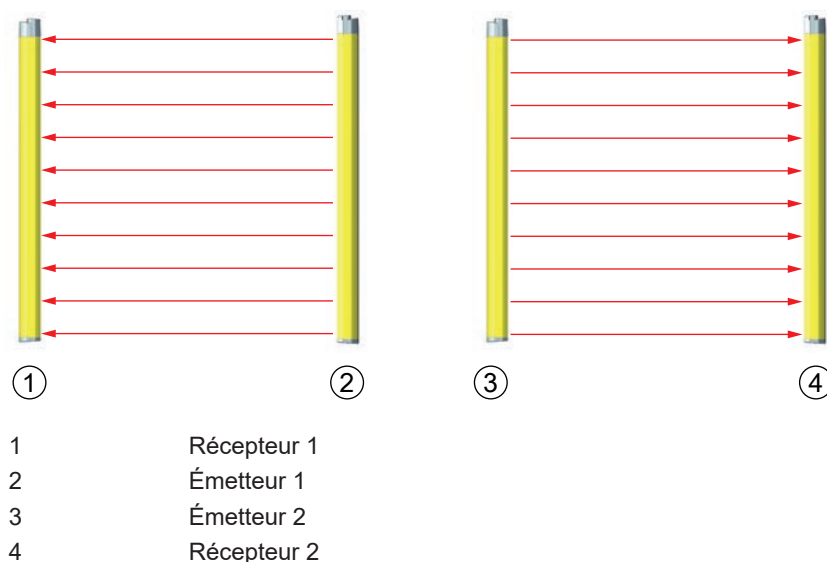
Fig. 6.5: Montage dans le sens opposé
