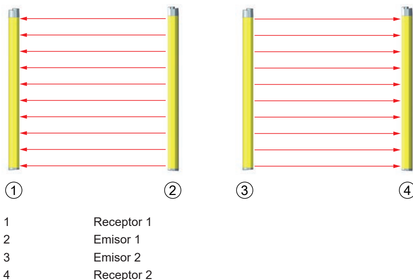
Figura 6.5: Montaje en sentido opuesto
