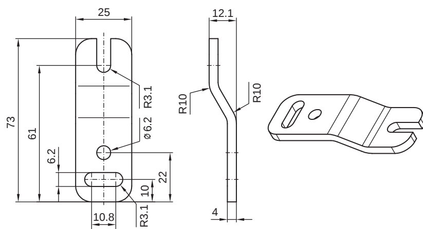
Bild 14.3: Parallelhalterung BT-Z
