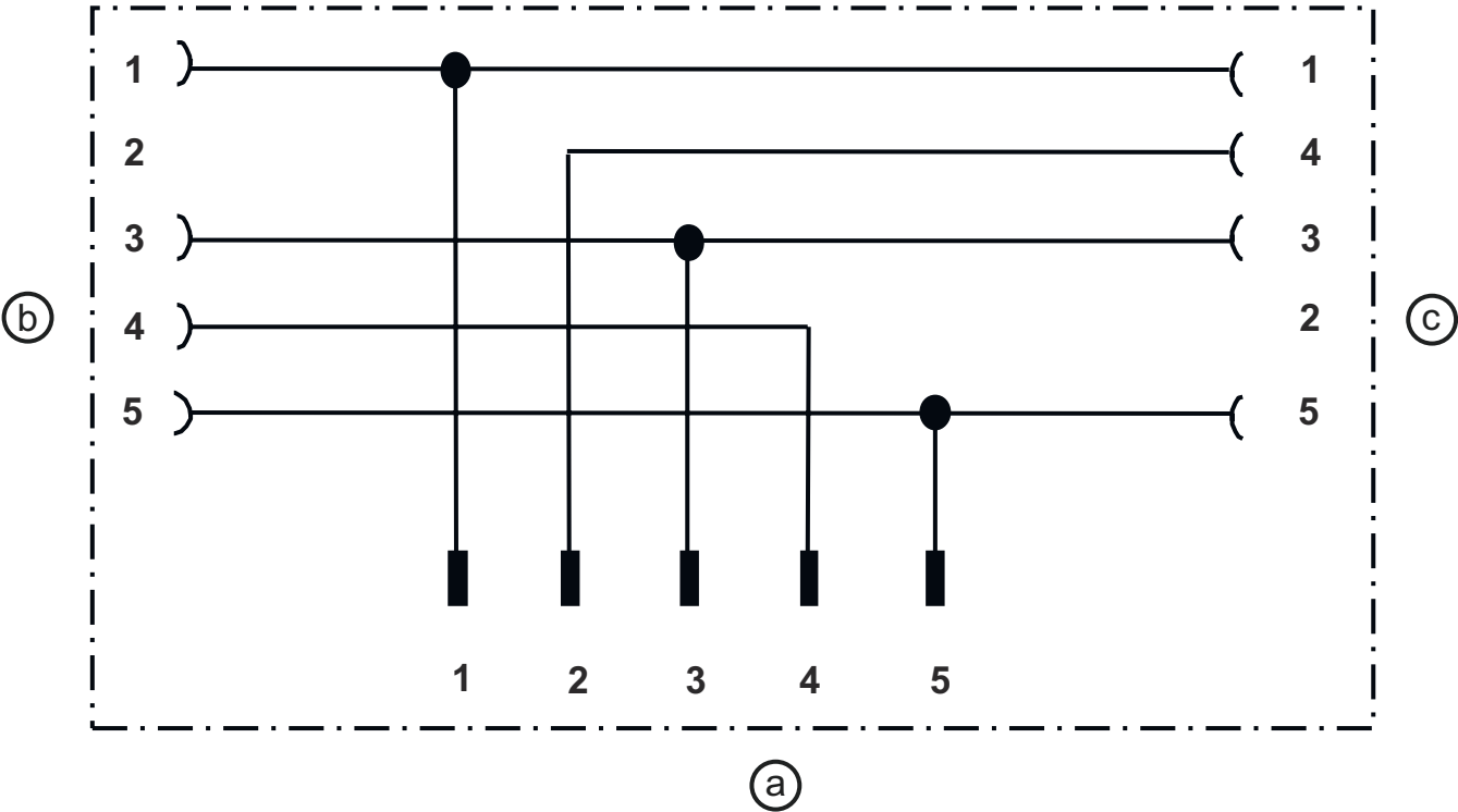
Diagrama de conexão
