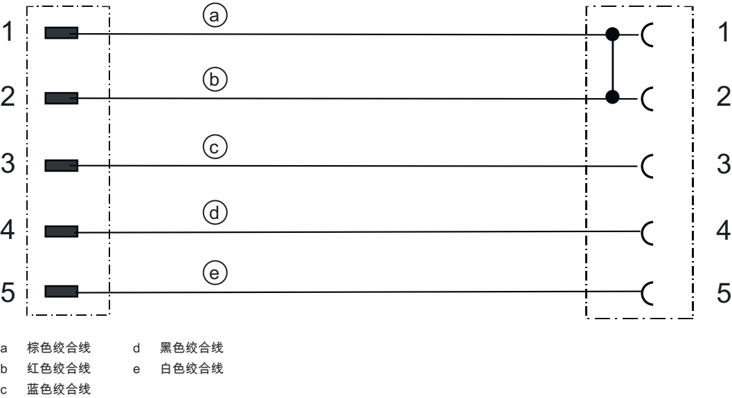
接线图
