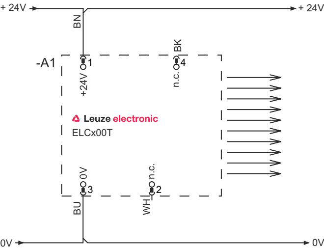
发射器连接图
