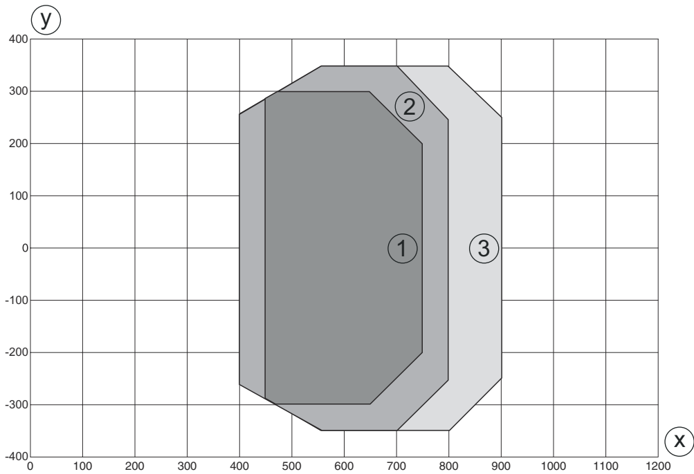
Curva del campo de lectura Medium Density
