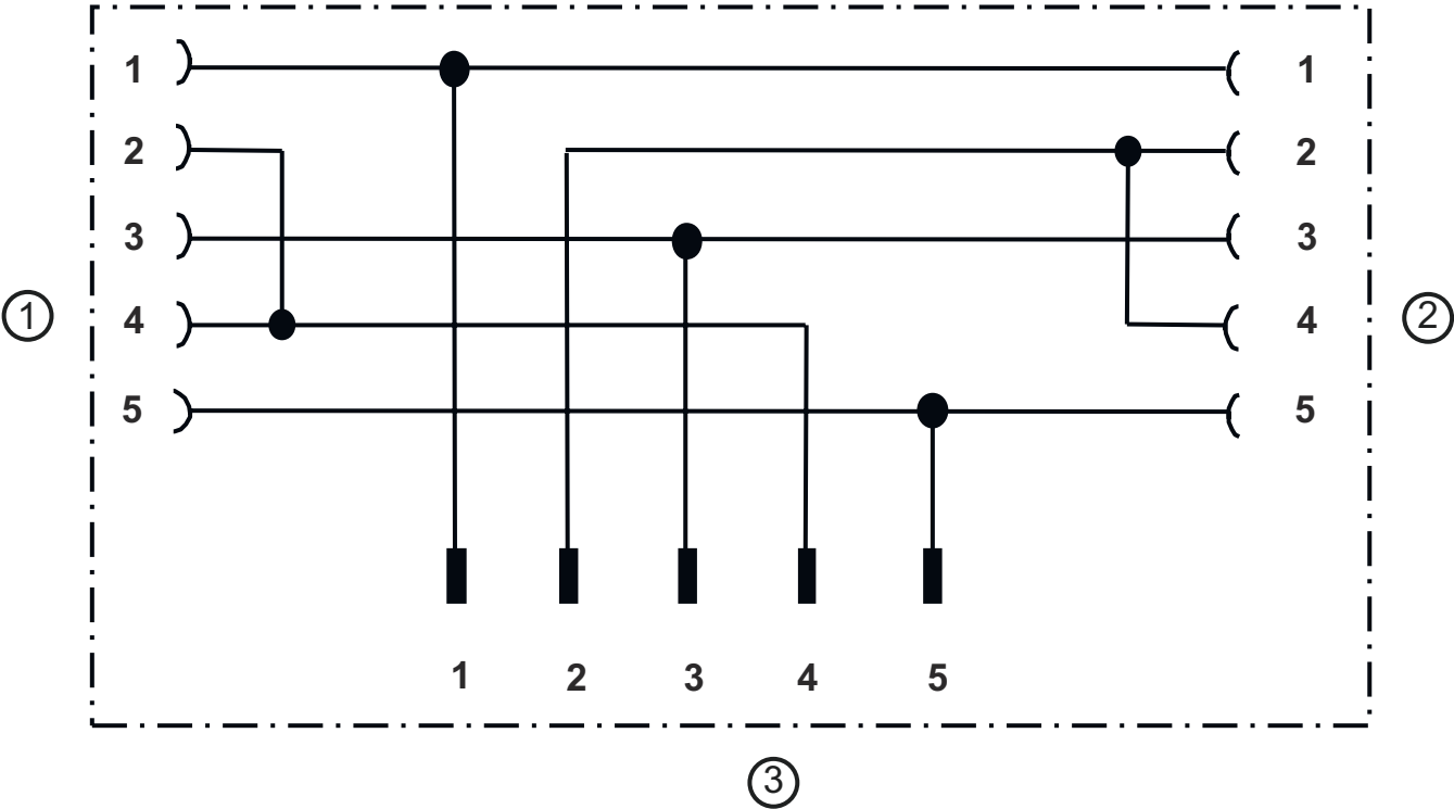
回線図
