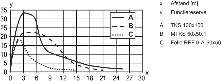
Typische functiereserve
