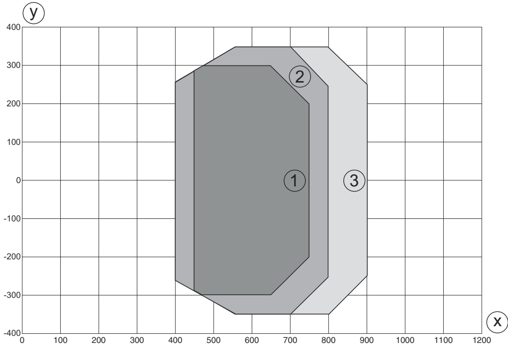
Curva do campo de leitura Medium Density
