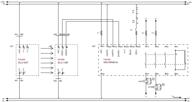
带后置安全控制器MSI-SR4B的接线示例
