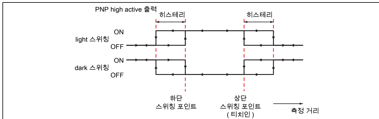
그림 3.6: ODSL 30/24... 스위칭 출력 상태 (PNP high active 출력)
