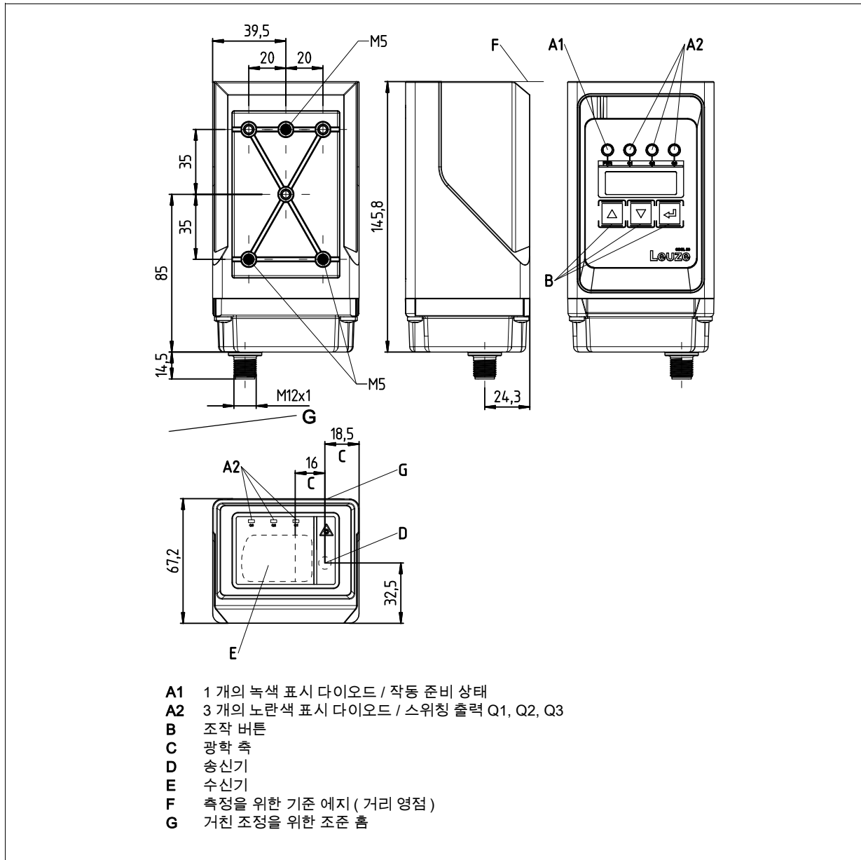
그림 4.1: 치수 도면 ODSL 30 - 유형
