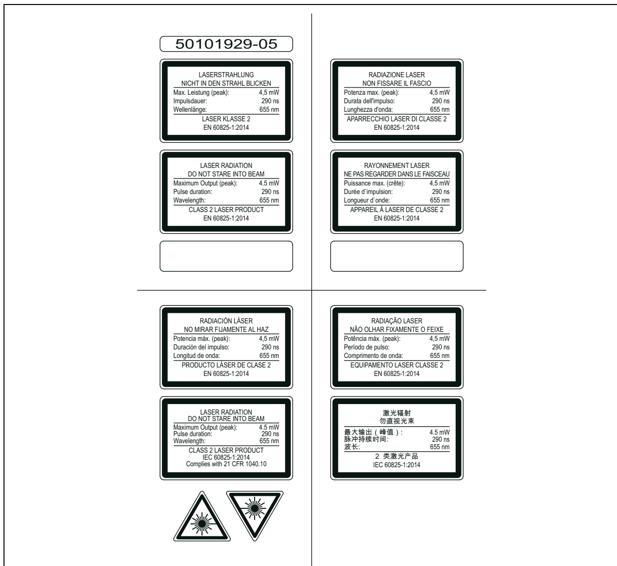
그림 2.2: 레이저 경고 라벨 및 레이저 주의 사항 라벨 - 동봉된 스티커
