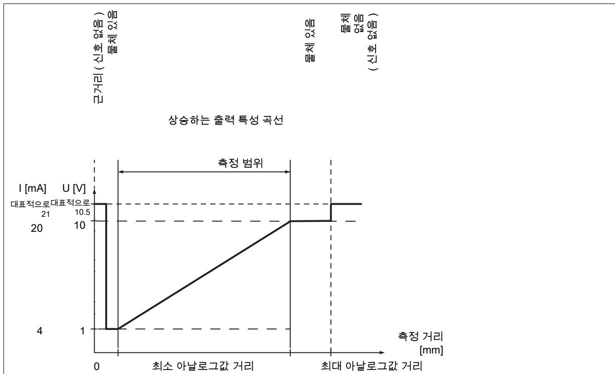
그림 3.4: 상승 곡선의 ODSL 30/V... 출력 특성 곡선
