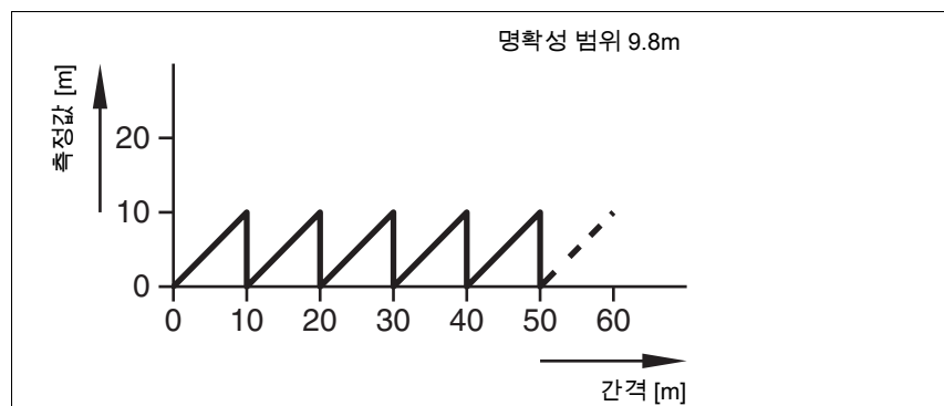
그림 3.10: 명확성 범위 9.8m 에서 ODSL 30 측정값
