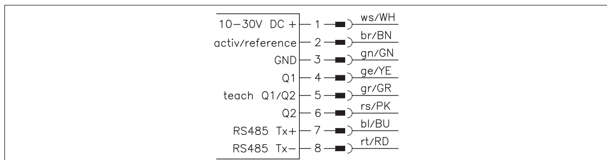
그림 4.5: ODSL 30/D 485... 전기 연결
