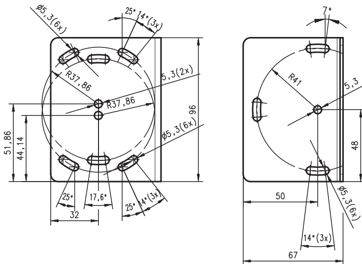
그림 3.3: BT 30 치수 도면
