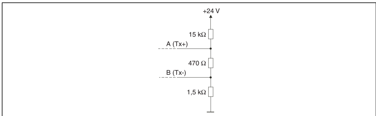
그림 3.8: RS 485 버스 종단용 분압기
