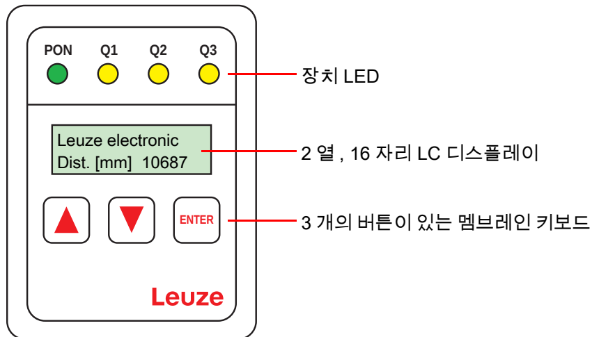
그림 3.9: ODSL 30 표시 및 조작 요소
