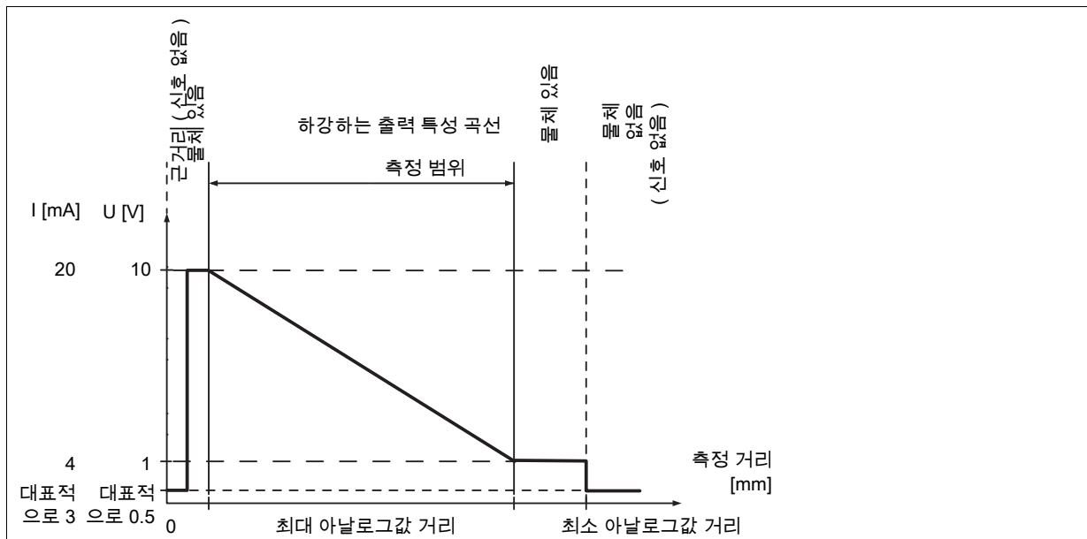
그림 3.5: 하강 곡선의 ODSL 30/V... 출력 특성 곡선
