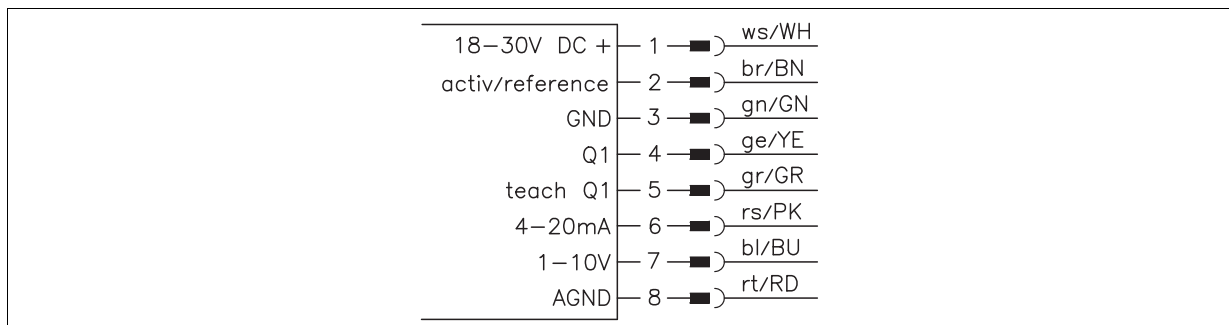
그림 4.2: ODSL 30/V... 전기 연결
