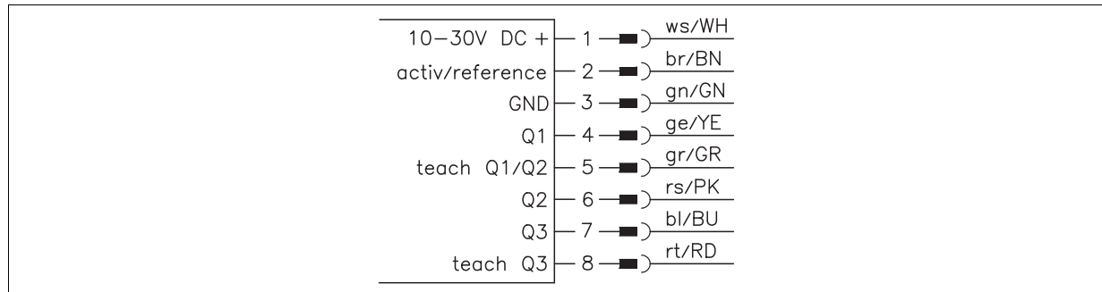
그림 4.3: ODSL 30/24... 전기 연결
