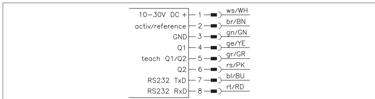
그림 4.4: ODSL 30/D 232... 전기 연결
