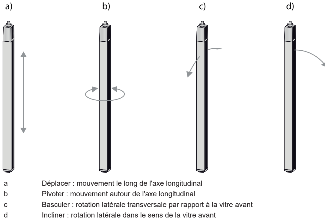
Fig. 5.6: Sens de déplacement pour l'alignement des rideaux lumineux
