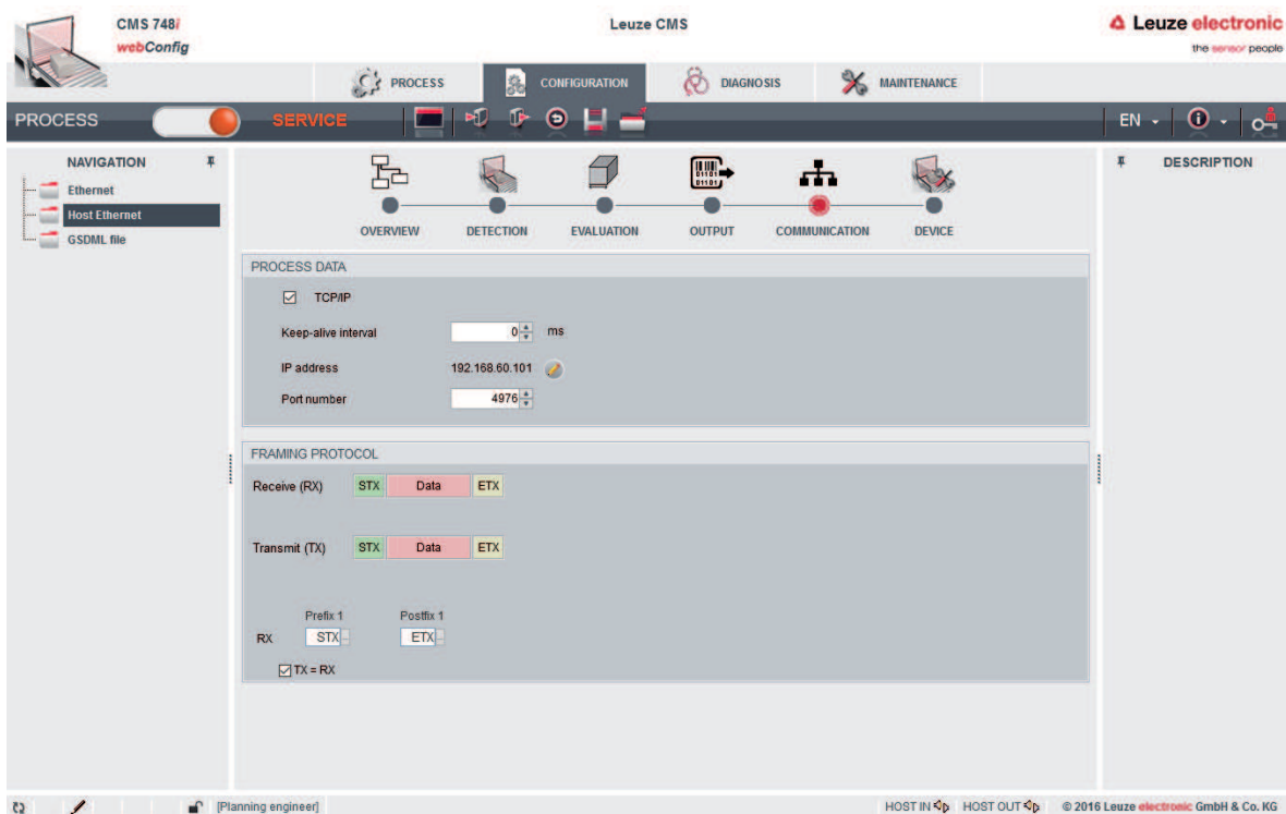
Fig. 8.11: Configuration de l'hôte Ethernet
