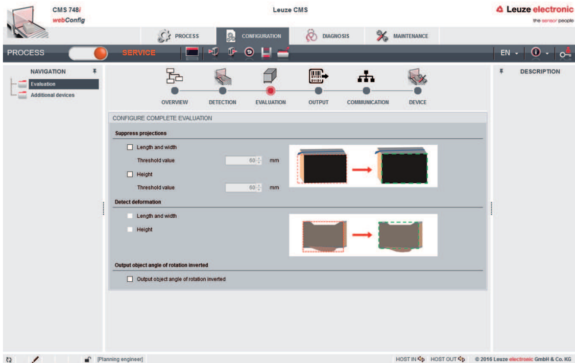
Fig. 8.8: Configuration de l'évaluation
