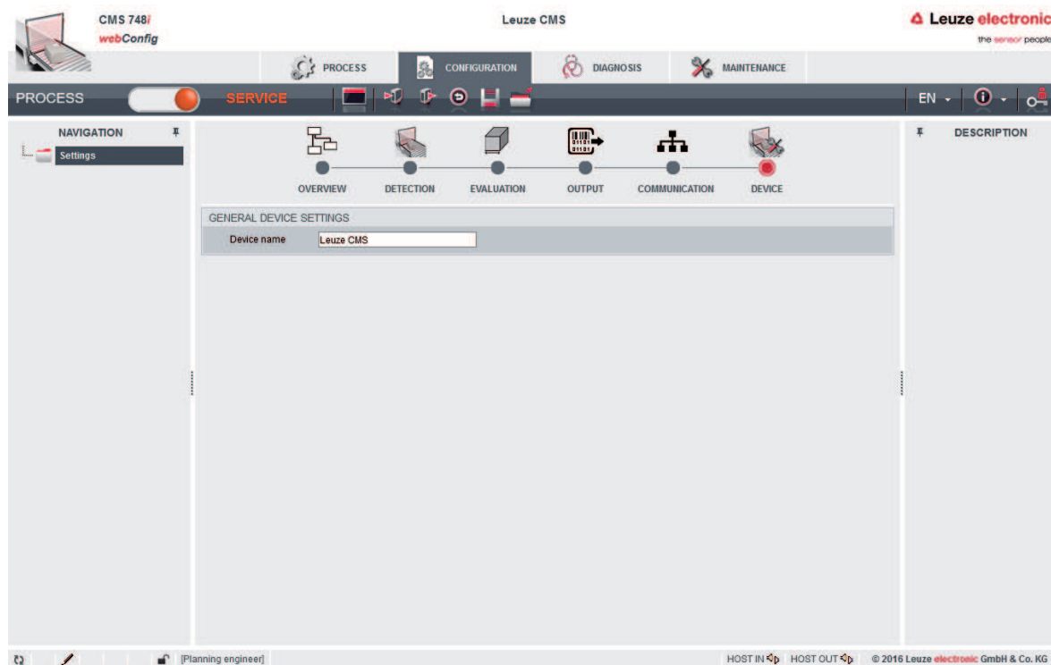
Fig. 8.12: Désignation du système de mesure des contours
