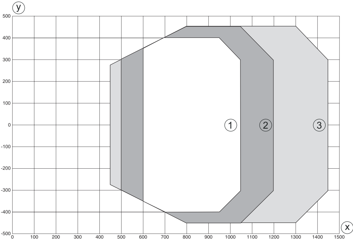
Curva del campo di lettura Low Density
