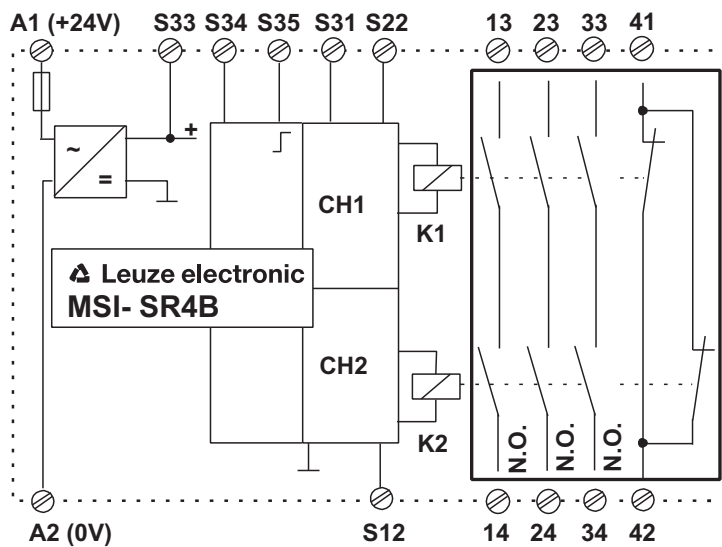
图 3.3: MSI-SR4B 的内部原理图
