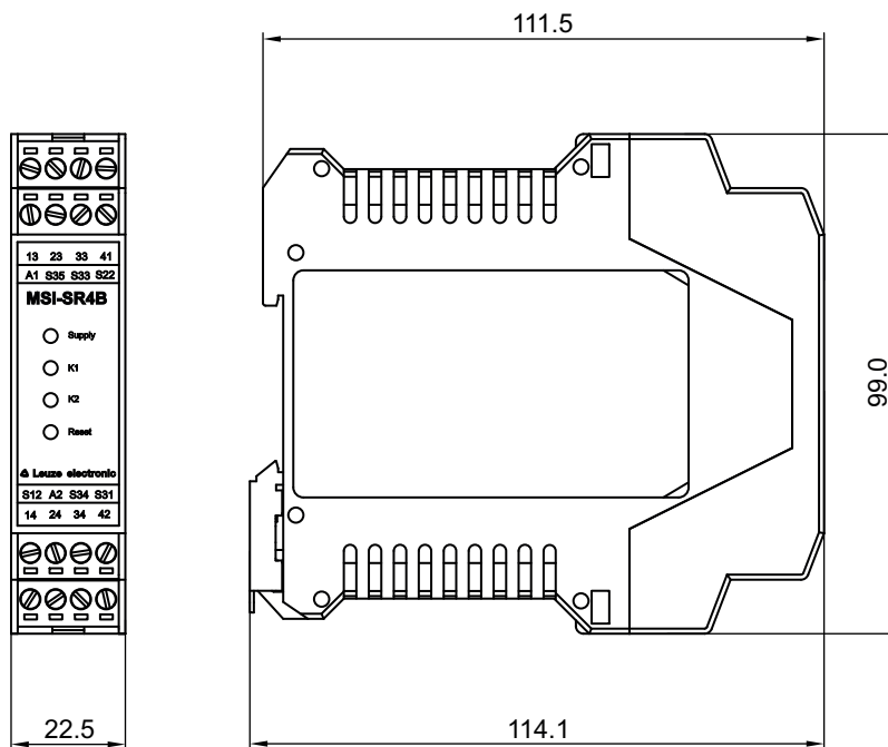
图 13.1: MSI-SR4B-01 尺寸
