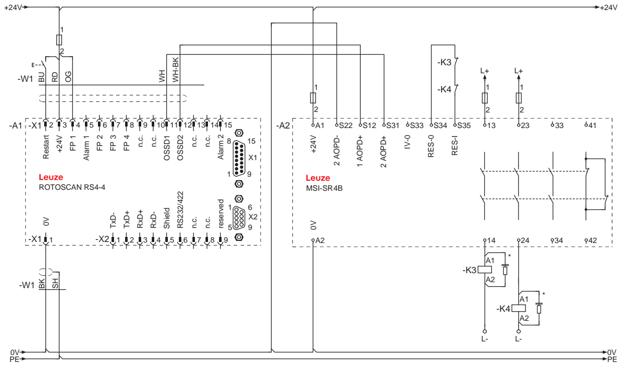
图 7.2: MSI-SR4B 相当于安全激光扫描仪 ROTOSCAN RS4-4 和带接触器监控 (EDM) 以及自动启动 / 重启功能 (通过激光扫描仪实现启动 / 重启联锁) 的机器控制系统之间的连接件
