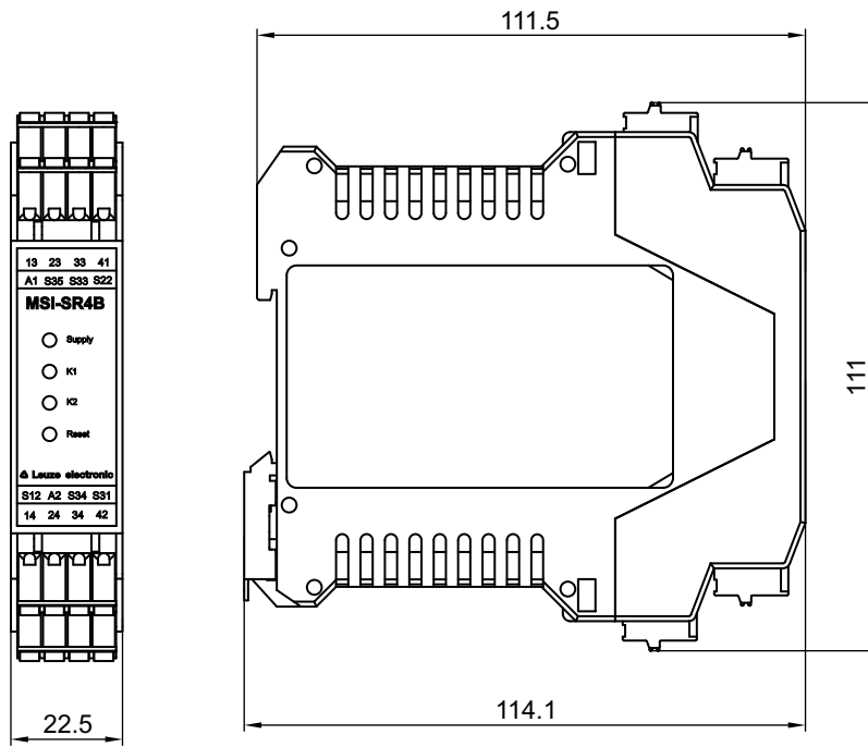
图 13.2: MSI-SR4B-02 尺寸
