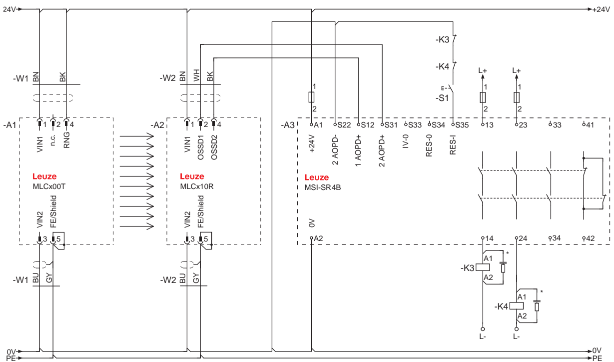
图 7.1: MSI-SR4B 与安全光幕 MLC 510
