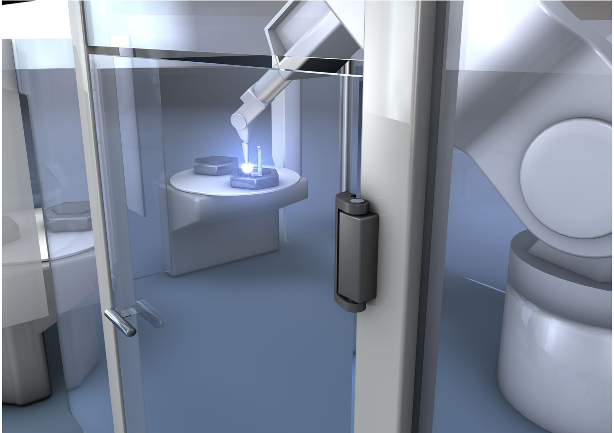
图 5.1: 通过安全铰链开关 S400 和安全继电器 MSI-SR4B 对机器人区域进行防护
